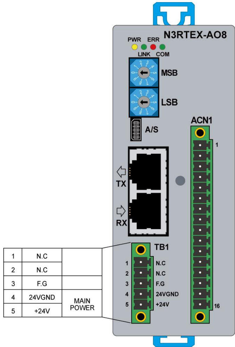
그림 41. N3RTEX-AO8 모듈 TB1 커넥터 핀 배열
