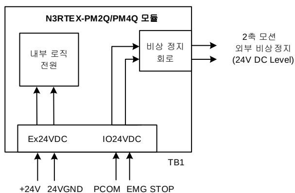
그림 73. N3RTEX-PM2Q/PM4Q 모듈 전원 회로 구성도
