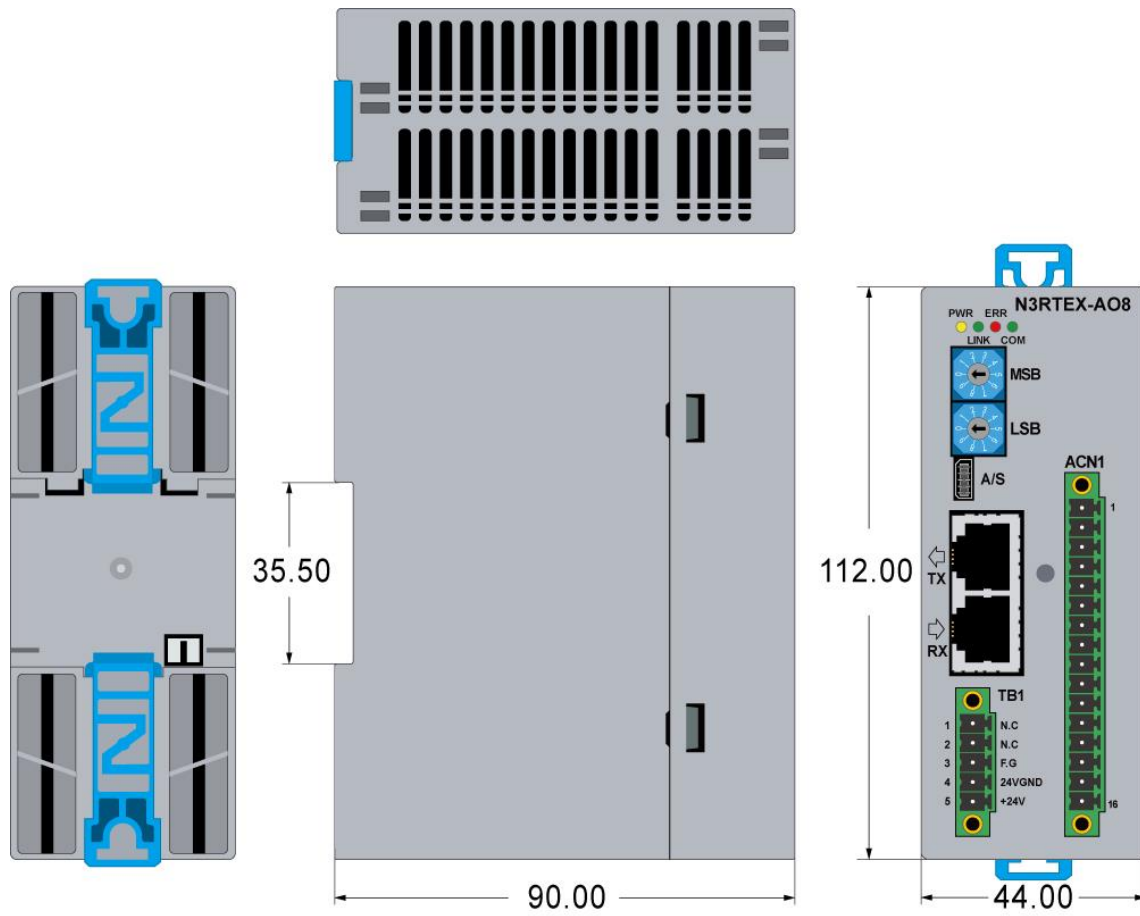
그림 9. N3RTEX-AO8 모듈의 사이즈 및 형상
