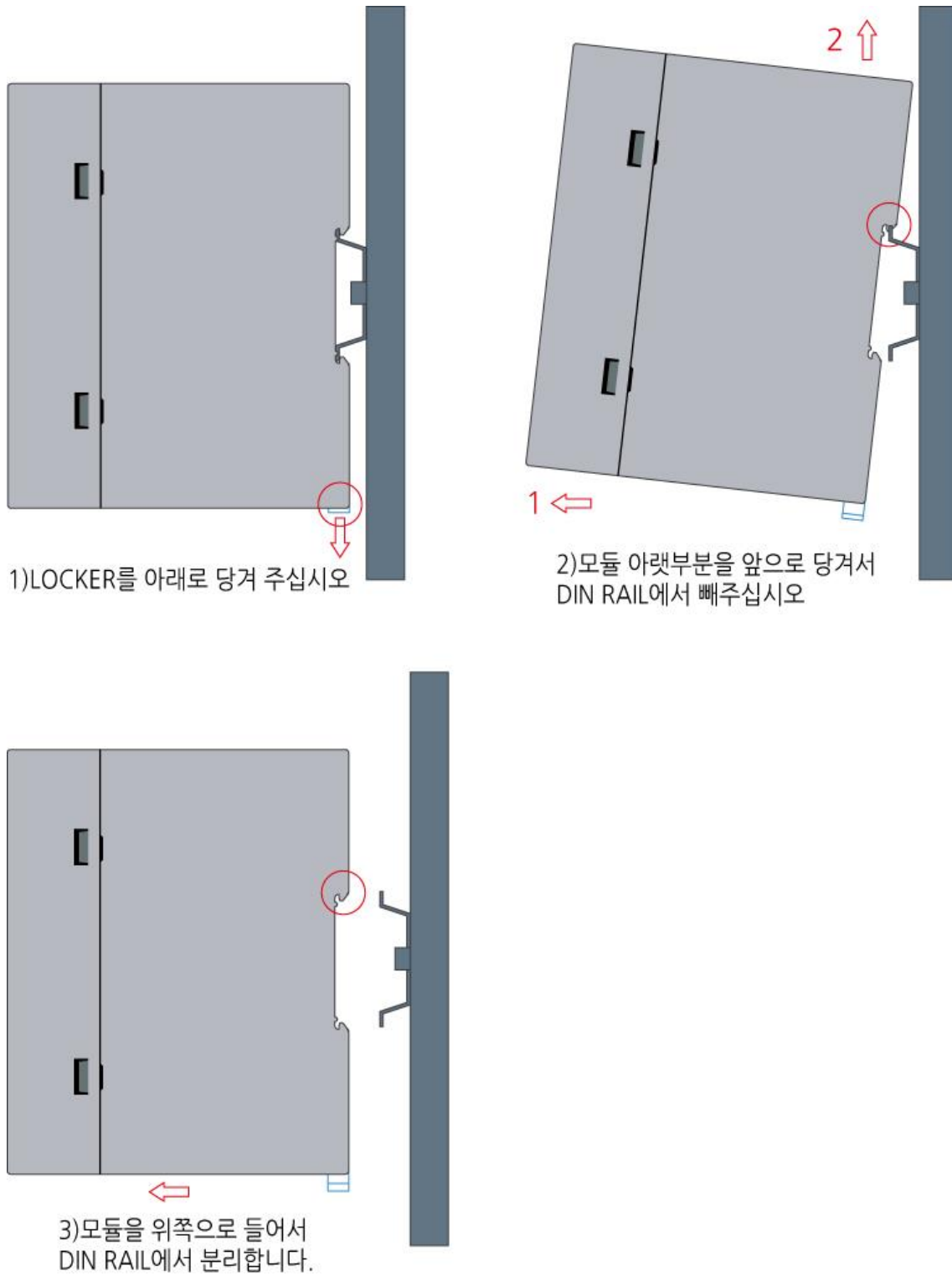
그림 15. 모듈 탈착 순서
