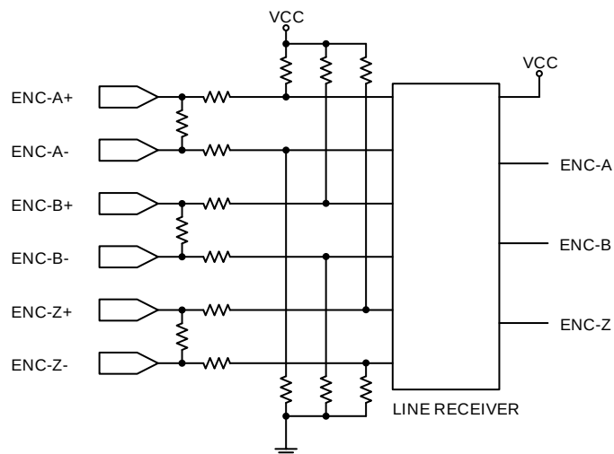
그림 74. N3RTEX-CNT2 모듈의 엔코더 입력 회로 구성도
