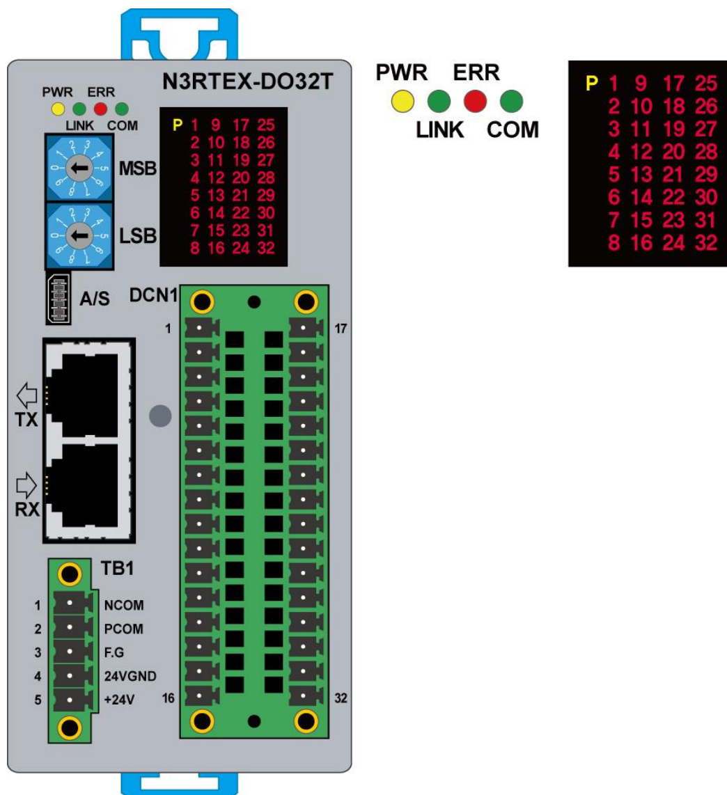
그림 22. N3RTEX-DO32T 모듈 LED 표시부
