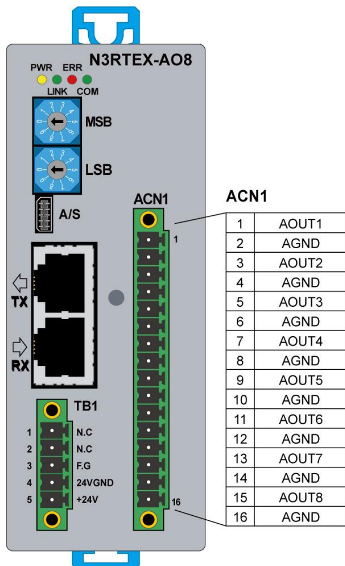
그림 37. N3RTEX-AO8 모듈 ACN1 커넥터 핀 배열
