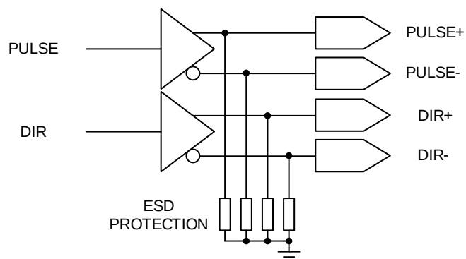
그림 67. N3RTEX-PM2Q/PM4Q 모듈의 펄스 출력 회로 구성도
