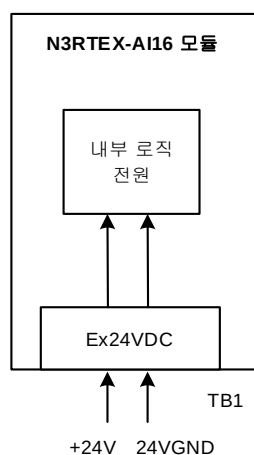
그림 64. N3RTEX-AI16 모듈 전원 회로 구성도
