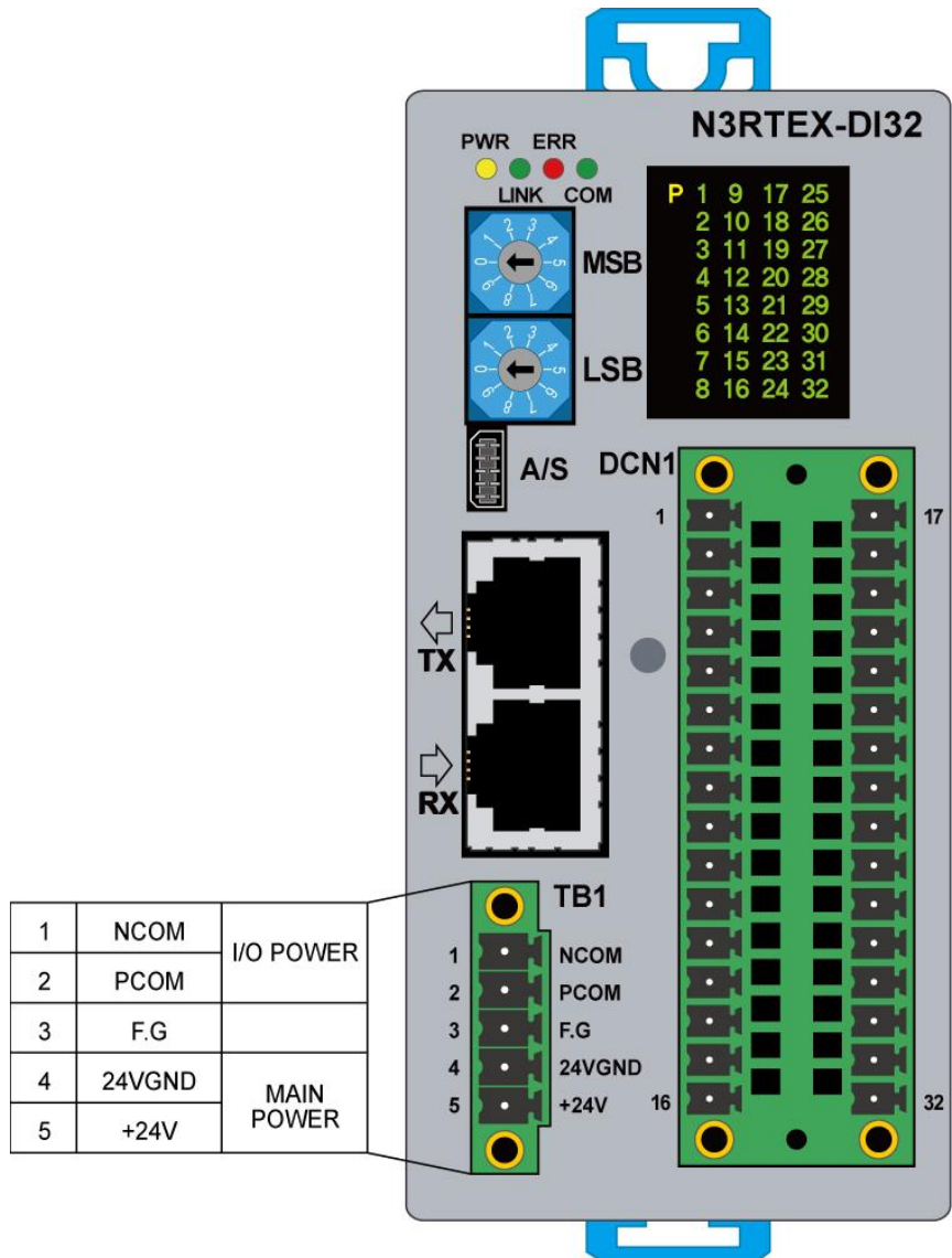
그림 20. N3RTEX-DI32 모듈 TB1 커넥터 핀 배열
