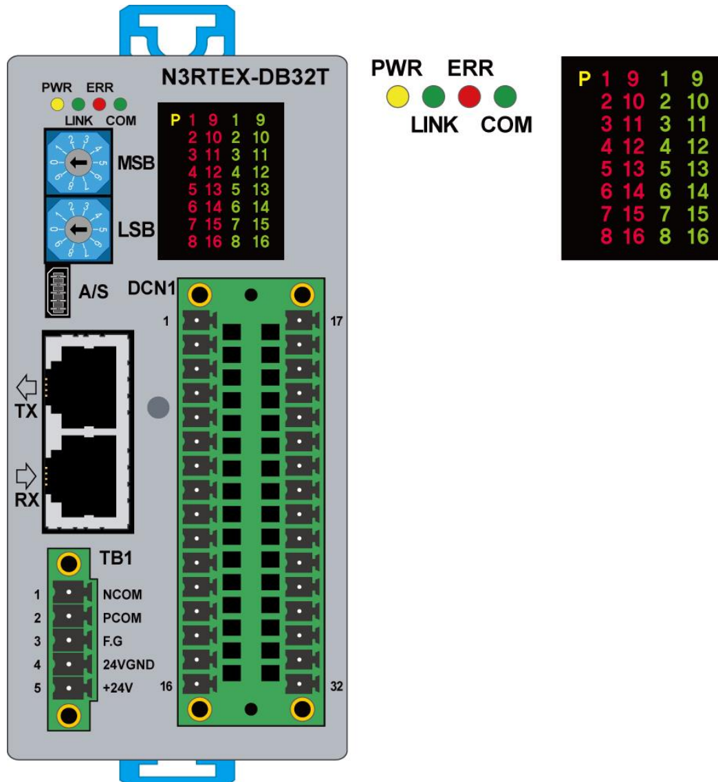
그림 27. N3RTEX-DB32T 모듈 LED 표시부
