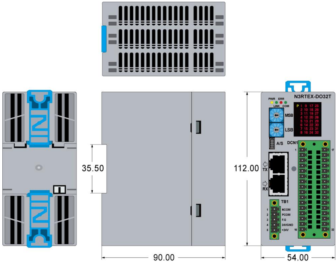
그림 6. N3RTEX-DO32T 모듈의 사이즈 및 형상
