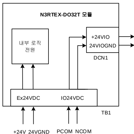
그림 60. N3RTEX-DO32T 모듈 전원 회로 구성도
