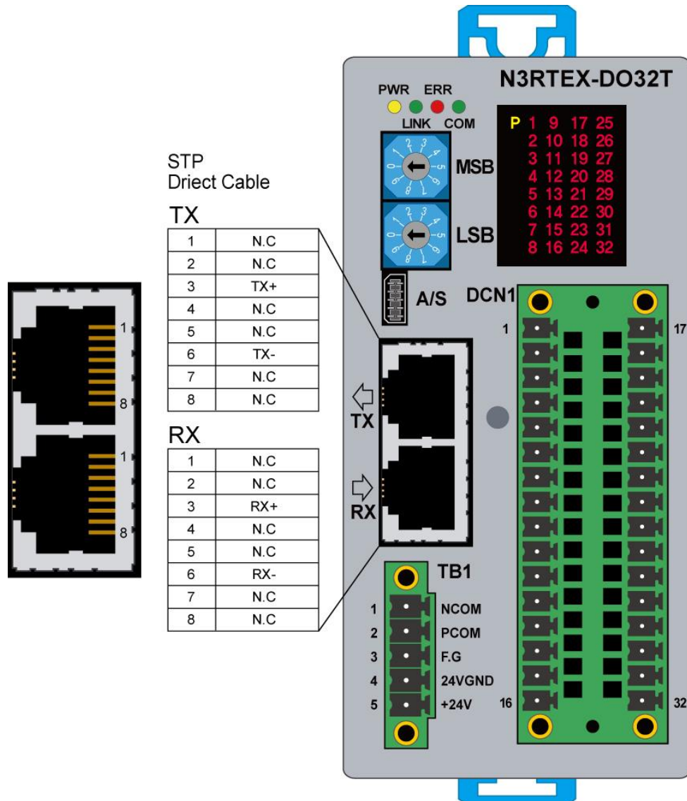
그림 24. N3RTEX-DO32T 모듈 RTEX 통신 커넥터 핀 배열 (RX, TX)
