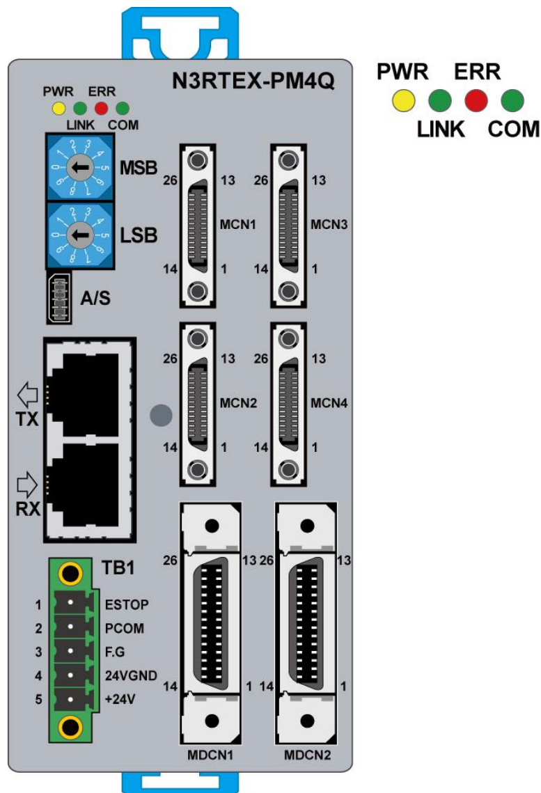
그림 48. N3RTEX-PM4Q 모듈 LED 표시부
