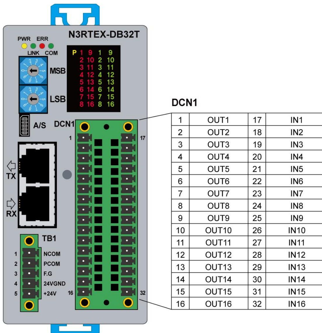
그림 26. N3RTEX-DB32T 모듈 DCN1 커넥터 핀 배열
