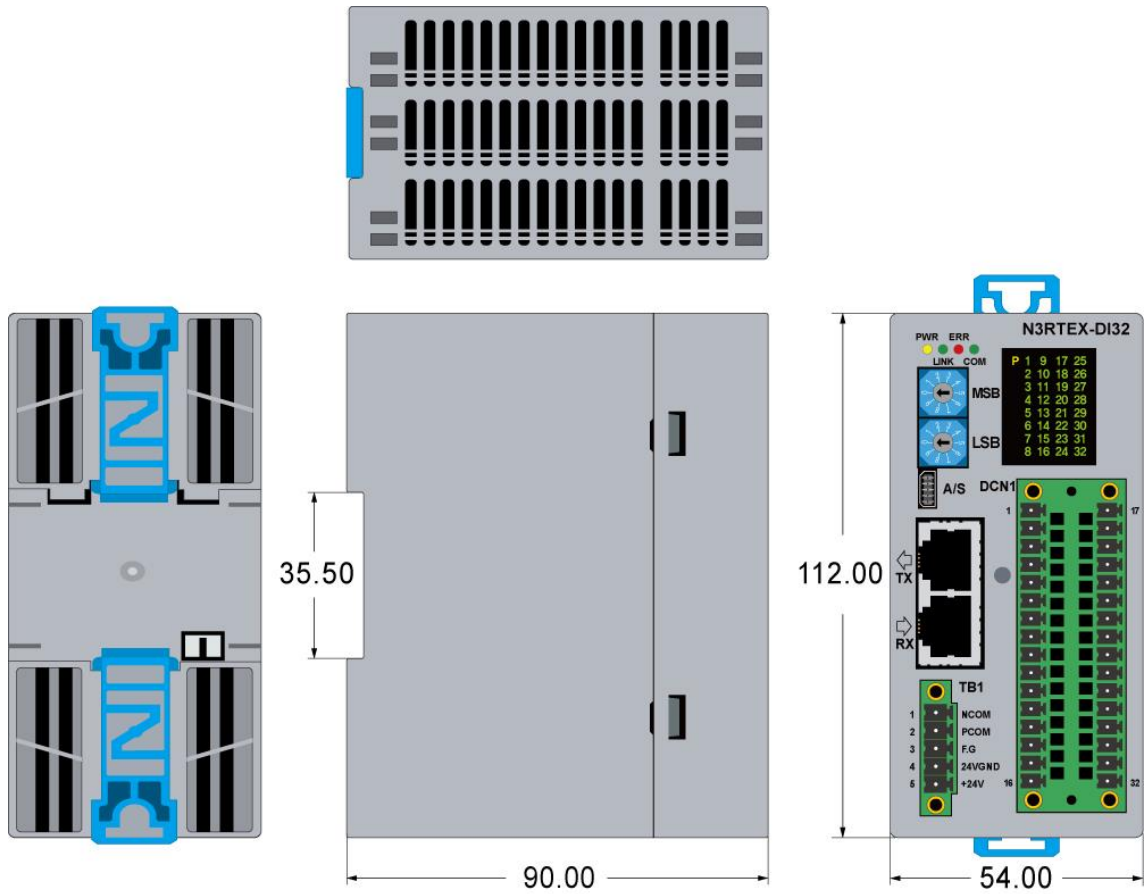
그림 5. N3RTEX-DI32 모듈의 사이즈 및 형상
