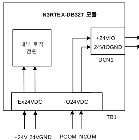
그림 62. N3RTEX-DB32T 모듈 전원 회로 구성도
