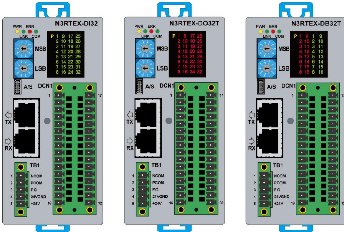
그림 1. N3 RTEX DIO SLAVE 모듈
