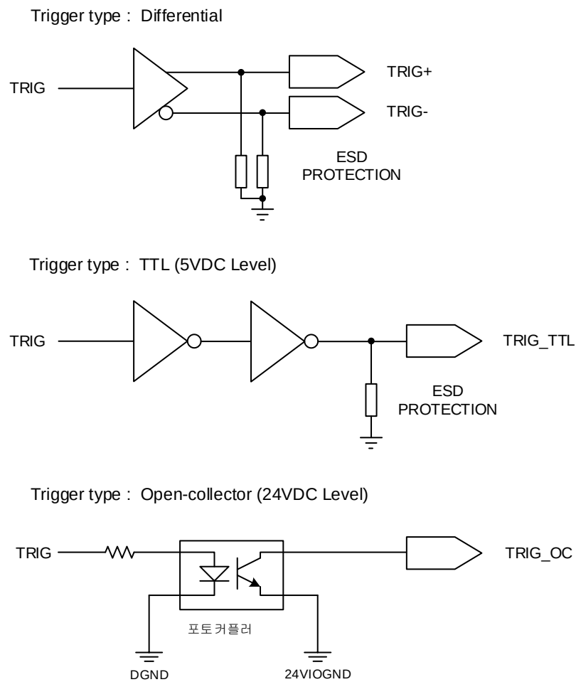
그림 75. N3RTEX-CNT2 모듈의 Trigger 회로 구성도
