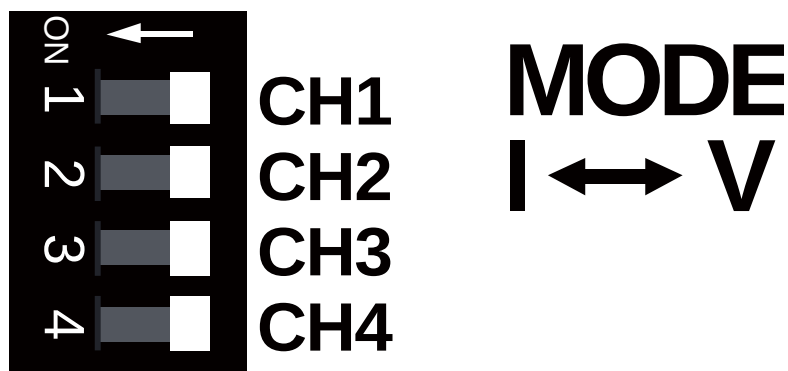
그림 33. N3RTEX-AI16 모듈 입력모드 스위치
