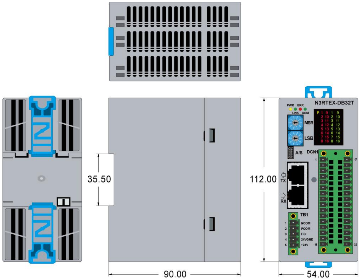
그림 7. N3RTEX-DB32T 모듈의 사이즈 및 형상
