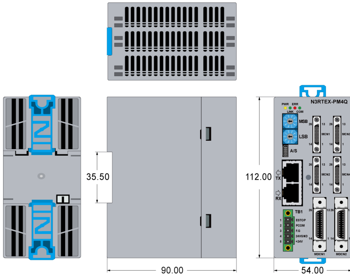
그림 11. N3RTEX-PM4Q 모듈의 사이즈 및 형상
