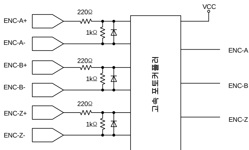
그림 68. N3RTEX-PM2Q/PM4Q 모듈 엔코더 입력 회로 구성도
