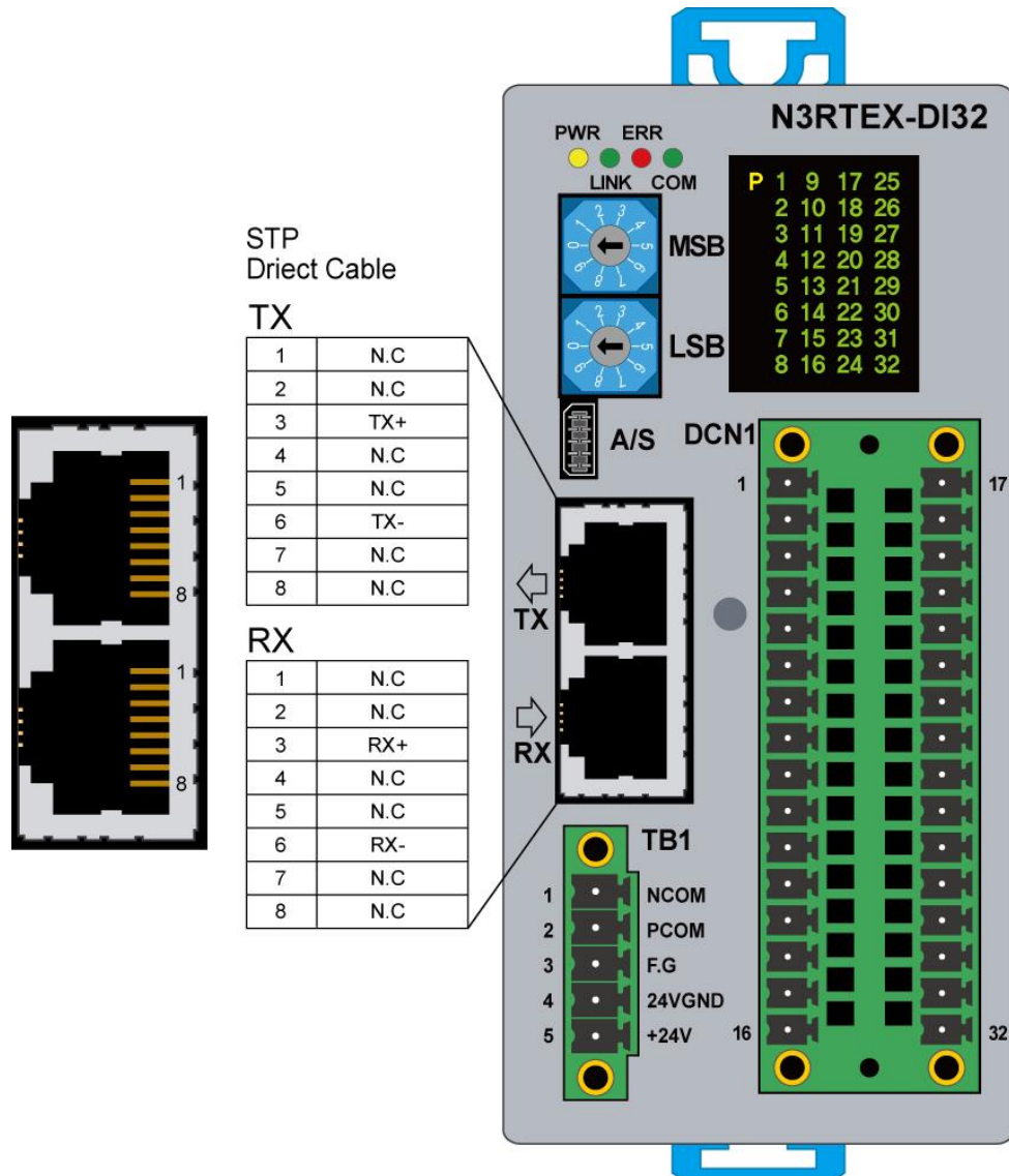
그림 19. N3RTEX-DI32 모듈 RTEX 통신 커넥터 핀 배열 (RX, TX)
