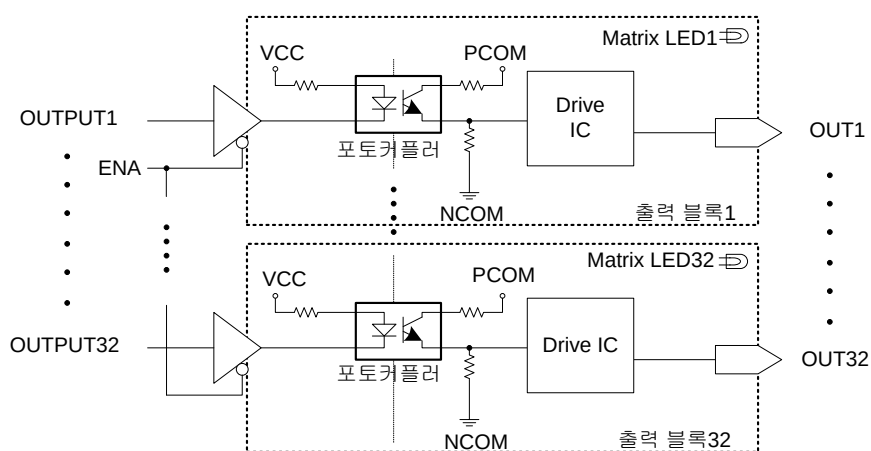
그림 59. N3RTEX-DO32T 모듈 내부의 디지털 출력 회로 구성도
