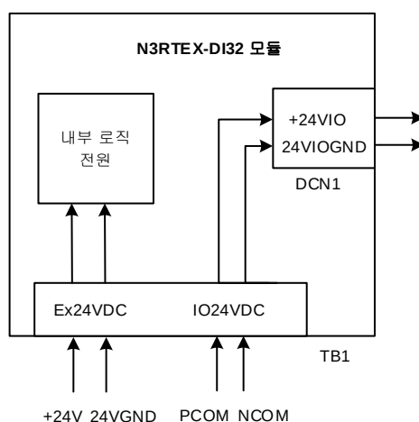
그림 58. N3RTEX-DI32 모듈 전원 회로 구성도
