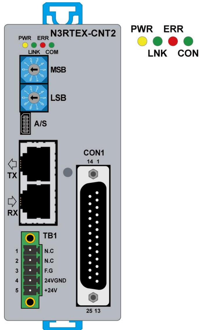
그림 53. N3RTEX-CNT2 모듈 LED 표시부
