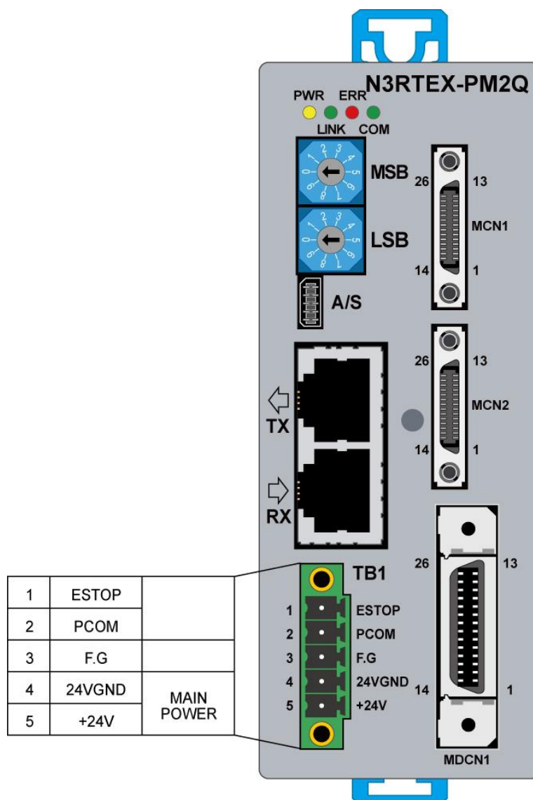
그림 46. N3RTEX-PM2Q 모듈 TB1 커넥터 핀 배열
