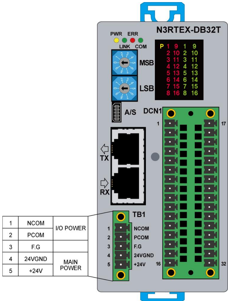
그림 30. N3RTEX-DB32T 모듈 TB1 커넥터 핀 배열
