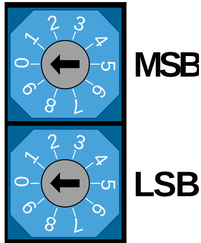
그림 23. N3RTEX-DO32T 모듈 NODE ID 스위치
