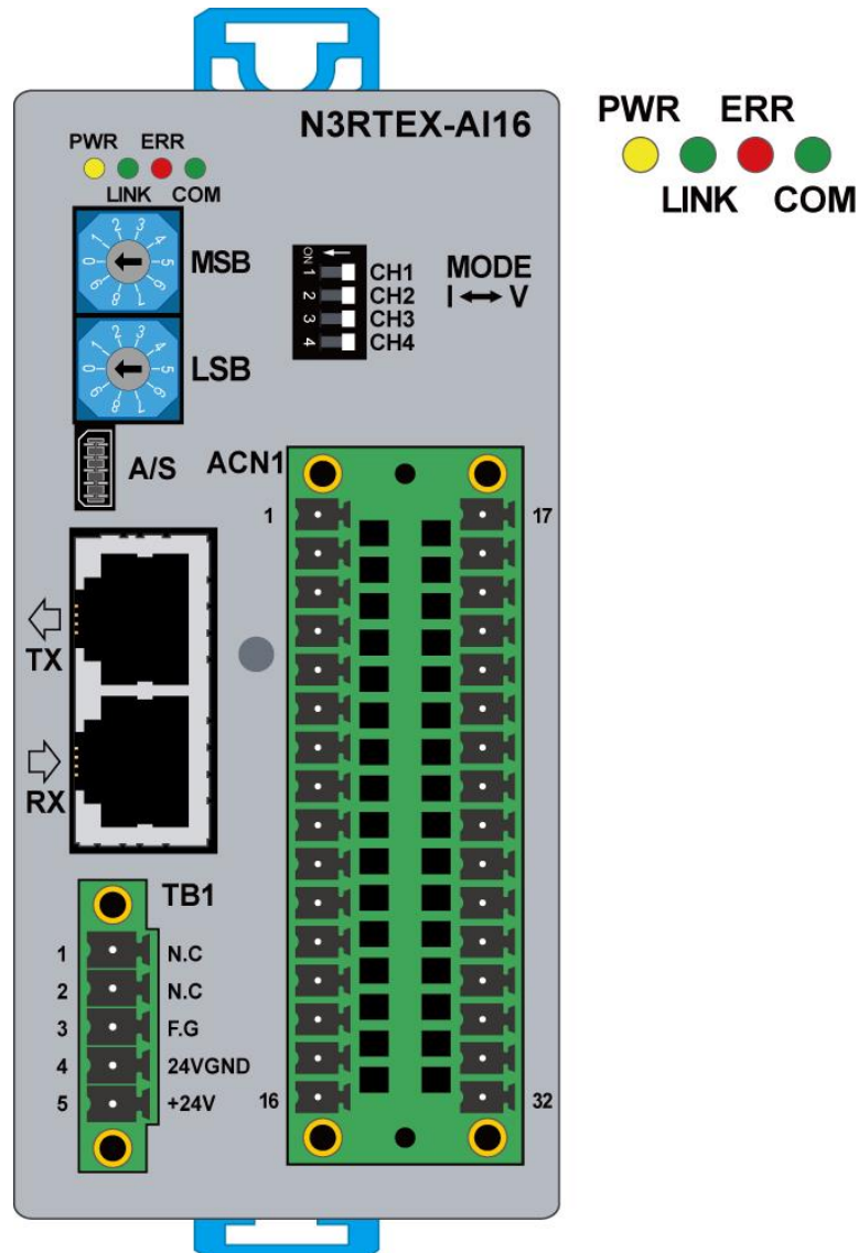
그림 32. N3RTEX-AI16 모듈 LED 표시부
