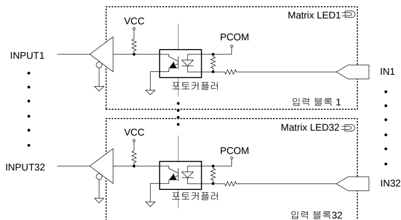
그림 57. N3RTEX-DI32 모듈 내부의 디지털 입력 회로 구성도
