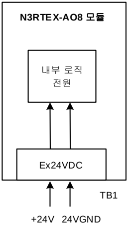
그림 66. N3RTEX-AO8 모듈 전원 회로 구성도
