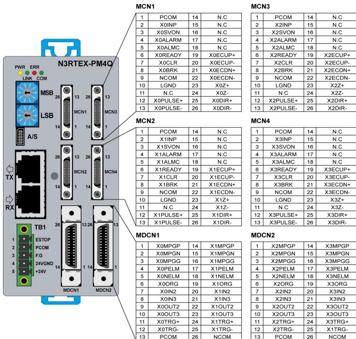
그림 47. N3RTEX-PM4Q의 MCN1~4, MDCN1~2 커넥터 핀 배열
