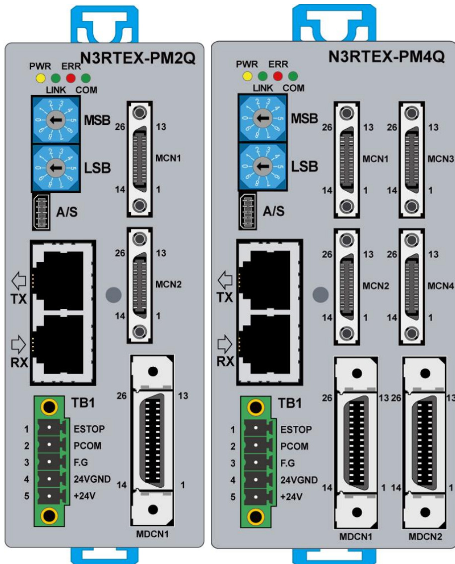
그림 3. N3RTEX PM2Q/PM4Q SLAVE 모듈
