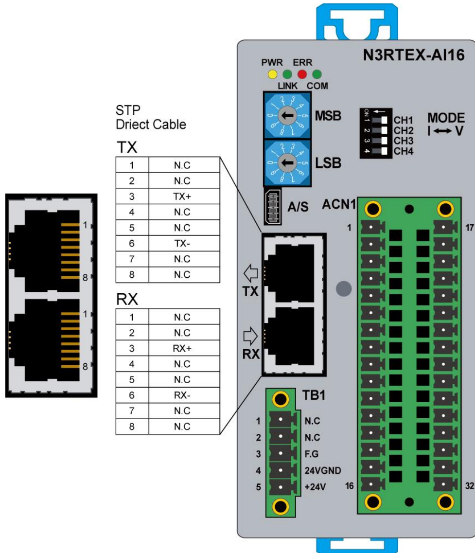
그림 35. N3RTEX-AI16 모듈 RTEX 통신 커넥터 핀 배열 (RX, TX)
