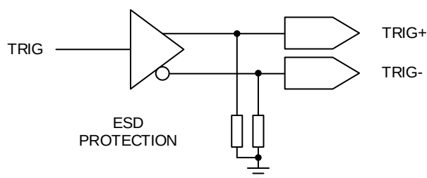
그림 71. N3RTEX-PM2Q/PM4Q 모듈의 TRIGGER 출력 회로 구성도
