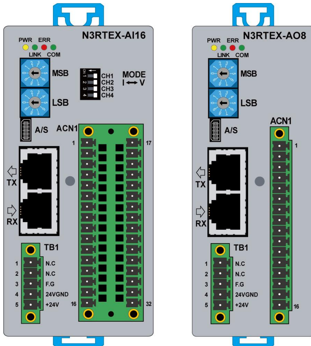
그림 2. N3 RTEX AIO SLAVE 모듈
