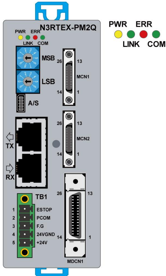
그림 43. N3RTEX-PM2Q 모듈 LED 표시부
