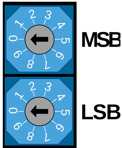
그림 44. N3RTEX-PM2Q 모듈 NODE ID 스위치
