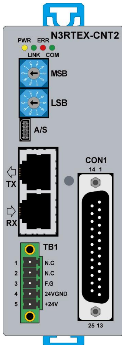
그림 4. N3RTEX CNT2 SLAVE 모듈
