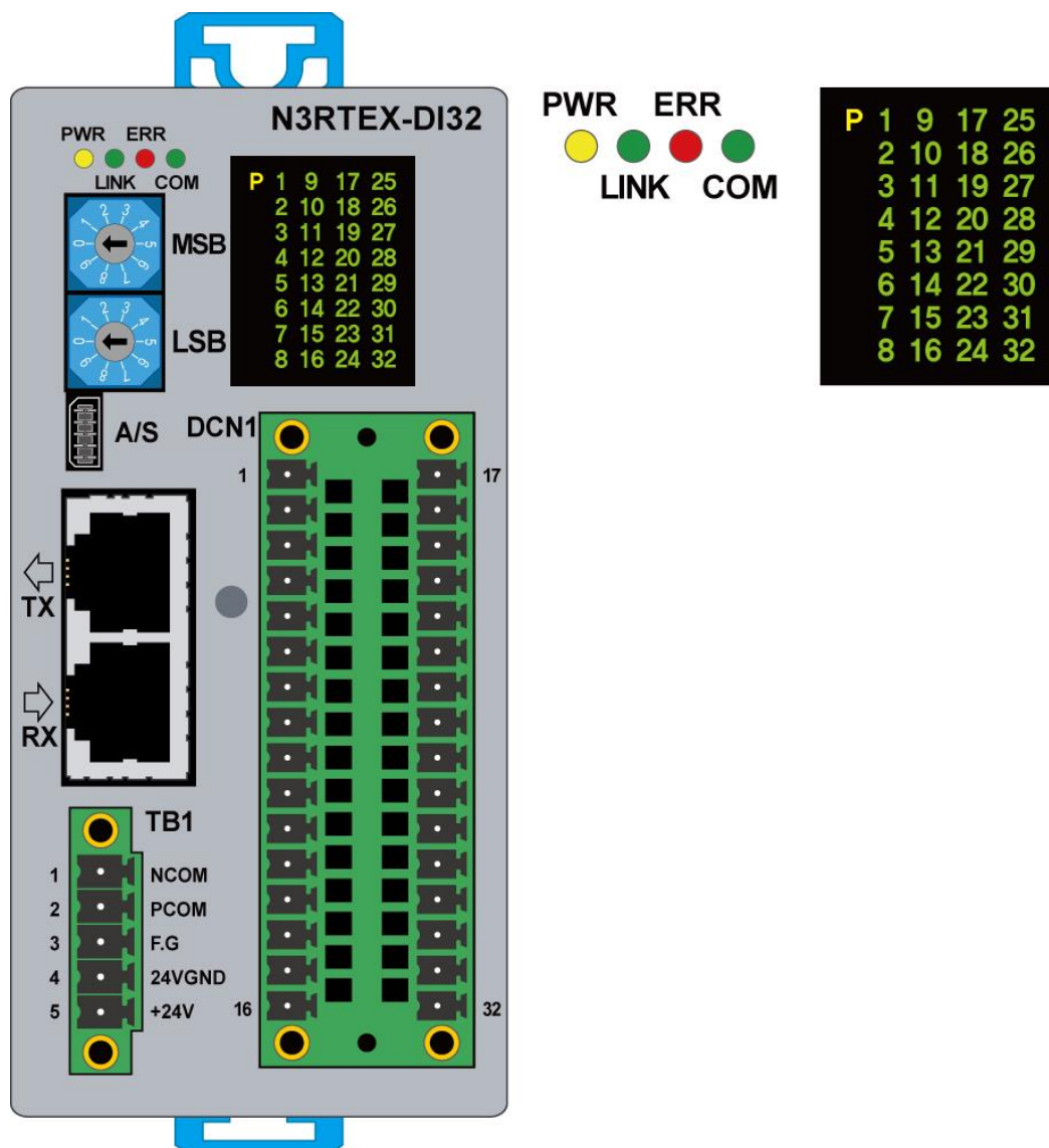
그림 17. N3RTEX-DI32 모듈 LED 표시부
