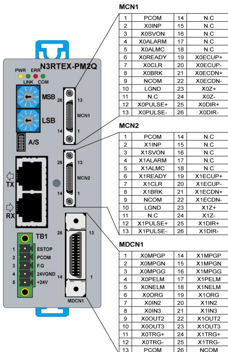
그림 42. N3RTEX-PM2Q의 MCN1, MCN2, MDCN1 커넥터 핀 배열
