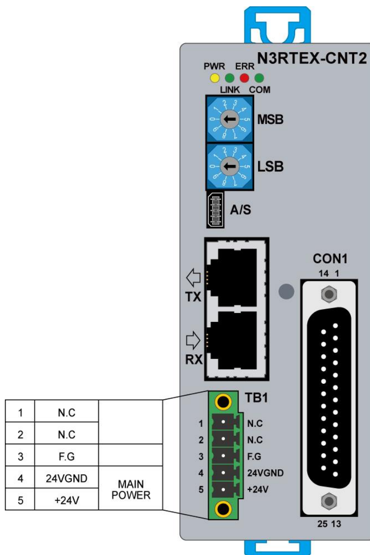
그림 56. N3RTEX-CNT2 모듈 TB1 커넥터 핀 배열
