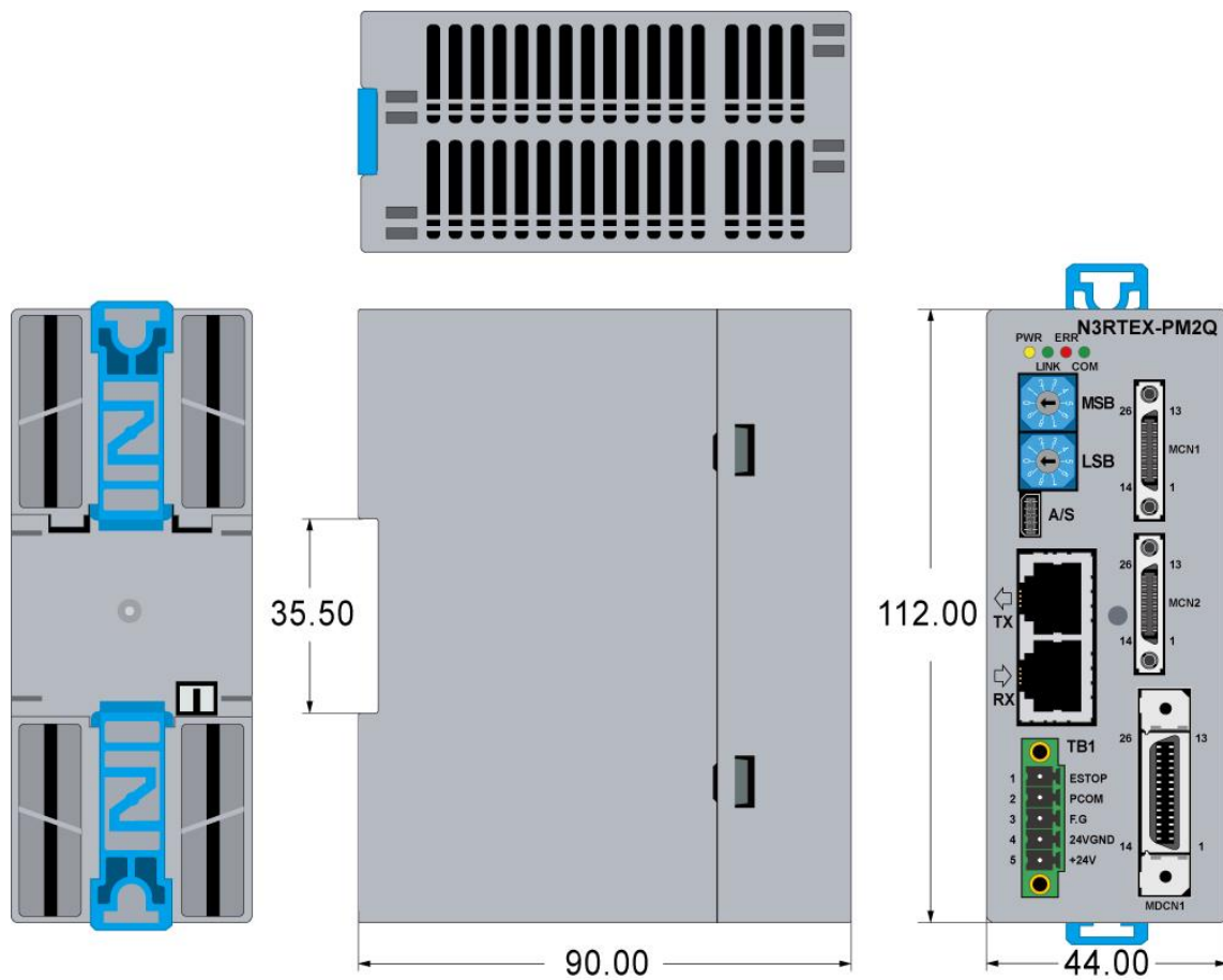
그림 10. N3RTEX-PM2Q 모듈의 사이즈 및 형상
