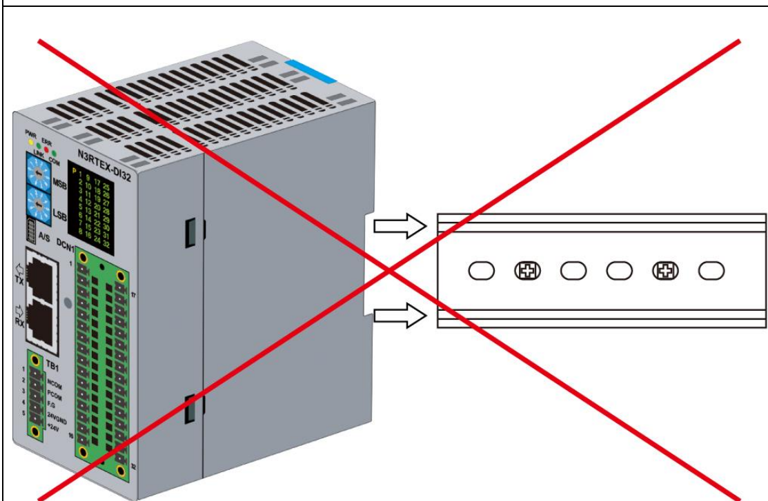
그림 13. DIN RAIL 측면 장착 금지
