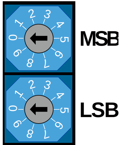
그림 18. N3RTEX-DI32 모듈 NODE ID 스위치
