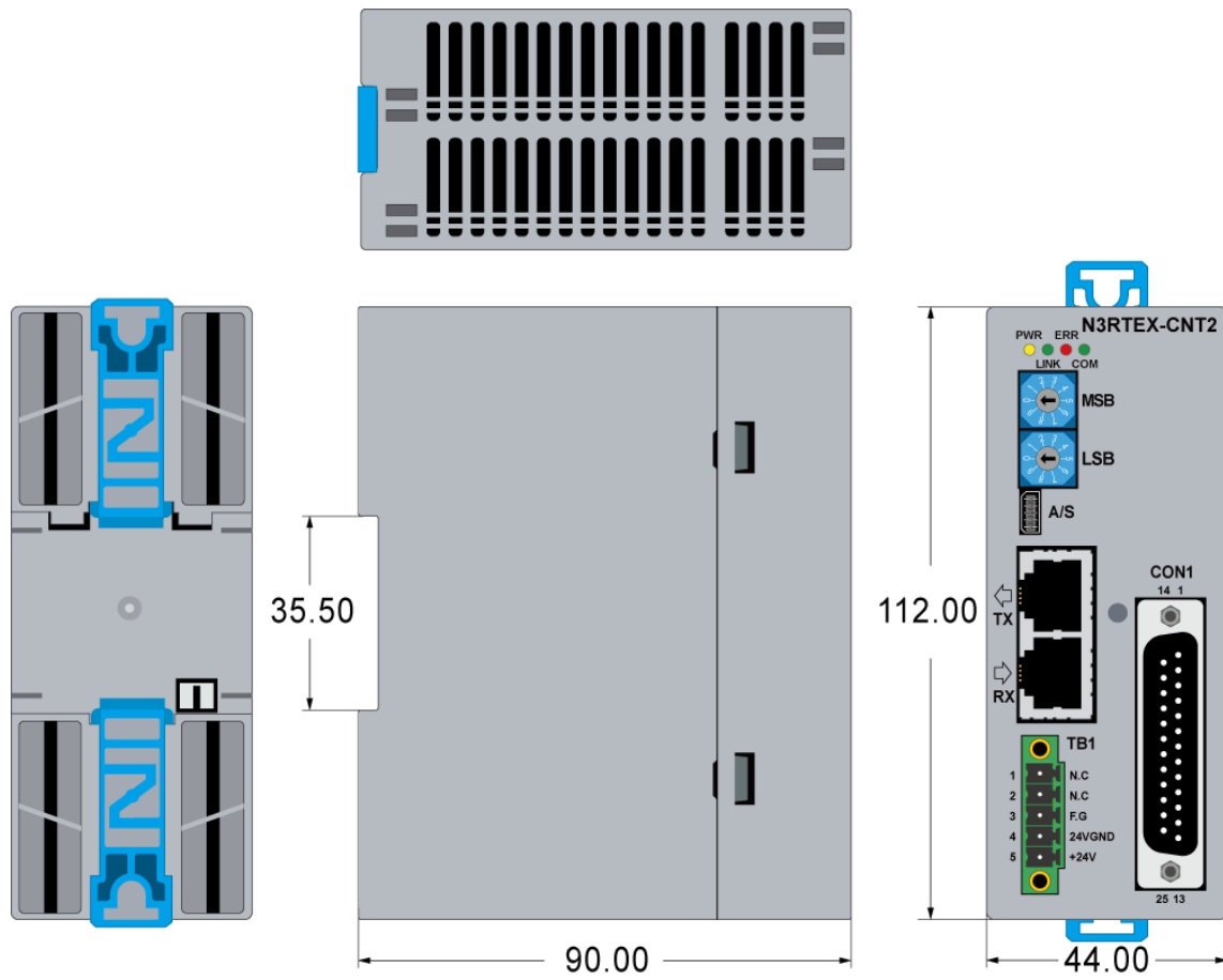
그림 12. N3RTEX-CNT2 모듈의 사이즈 및 형상
