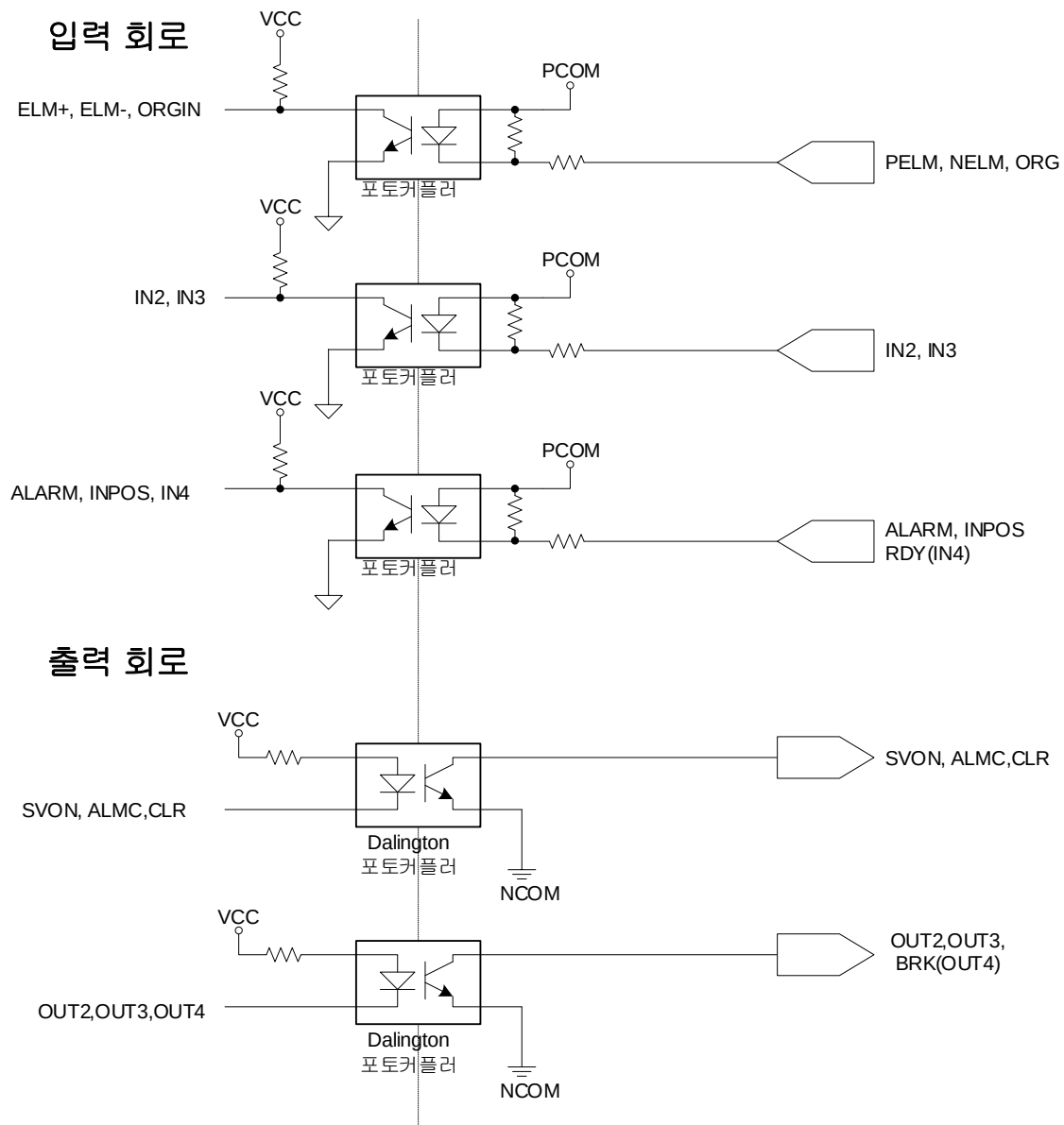
그림 69. N3RTEX-PM2Q/PM4Q 모듈의 모션 디지털 입력/출력 회로 구성도
