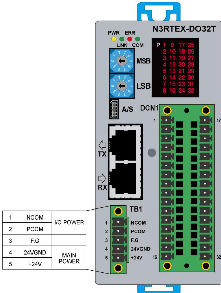
그림 25. N3RTEX-DO32T 모듈 TB1 커넥터 핀 배열
