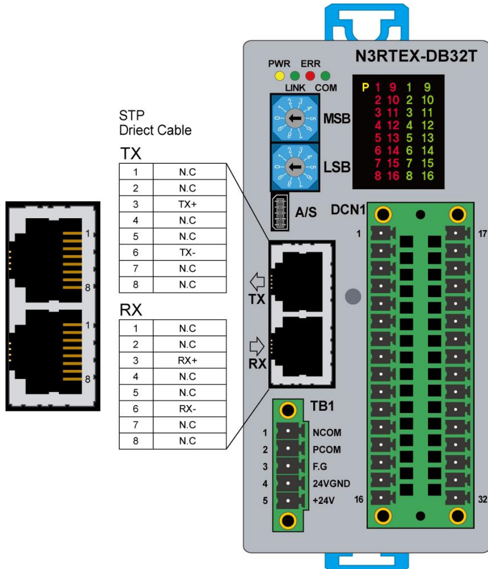
그림 29. N3RTEX-DB32T 모듈 RTEX 통신 커넥터 핀 배열 (RX, TX)
