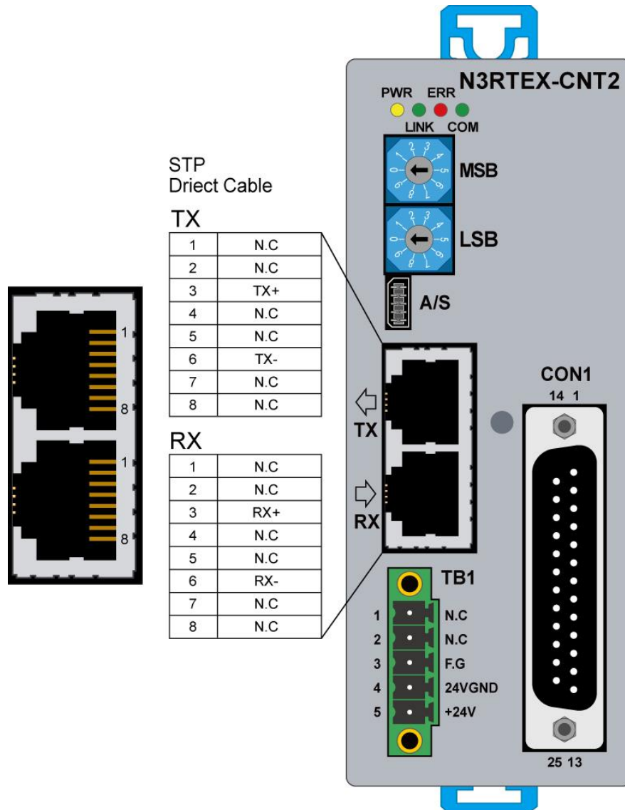
그림 55. N3RTEX-CNT2 모듈 RTEX 통신 커넥터 핀 배열 (RX, TX)
