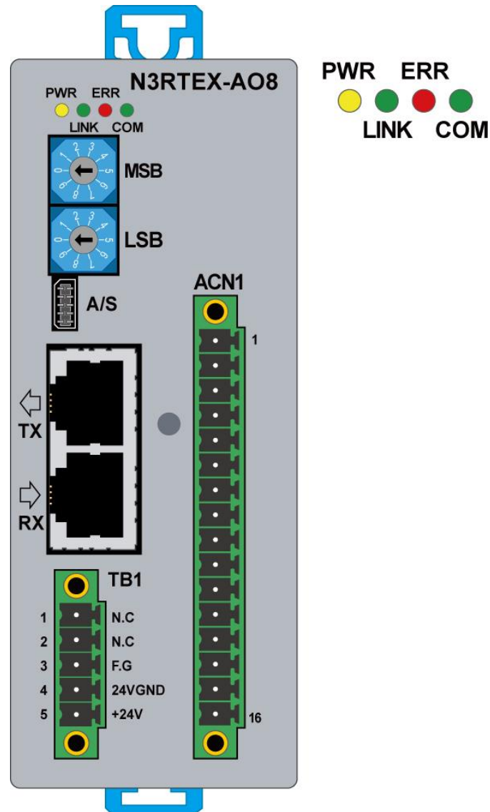
그림 38. N3RTEX-AO8 모듈 LED 표시부
