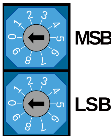
그림 34. N3RTEX-AI16 모듈 NODE ID 스위치
