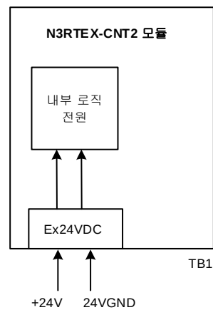
그림 76. N3RTEX-CNT2 모듈 전원 회로 구성도
