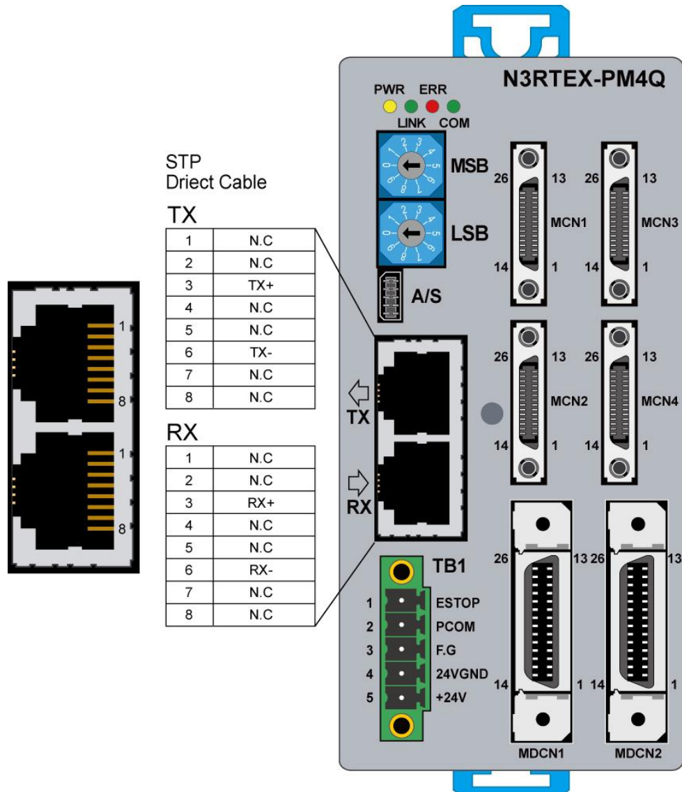
그림 50. N3RTEX-PM4Q 모듈 RTEX 통신 커넥터 핀 배열 (RX, TX)
