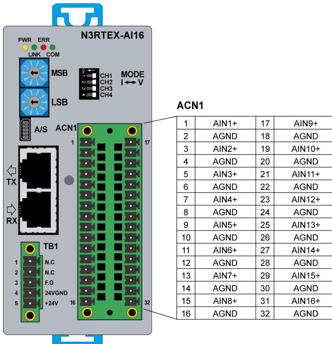
그림 31. N3RTEX-AI16 모듈 ACN1 커넥터 핀 배열
