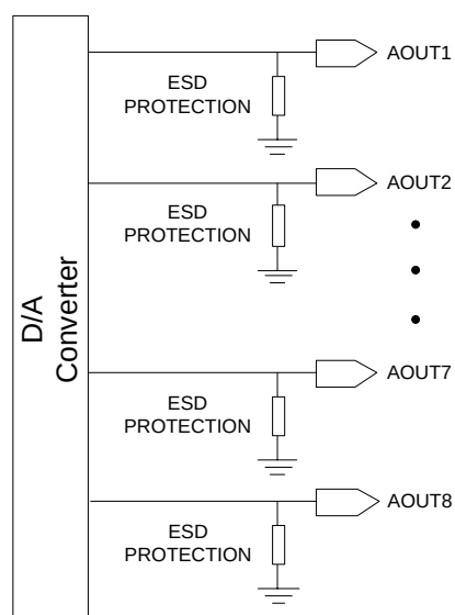
그림 65. N3RTEX-AO8 모듈 내부의 아날로그 출력 회로 구성도
