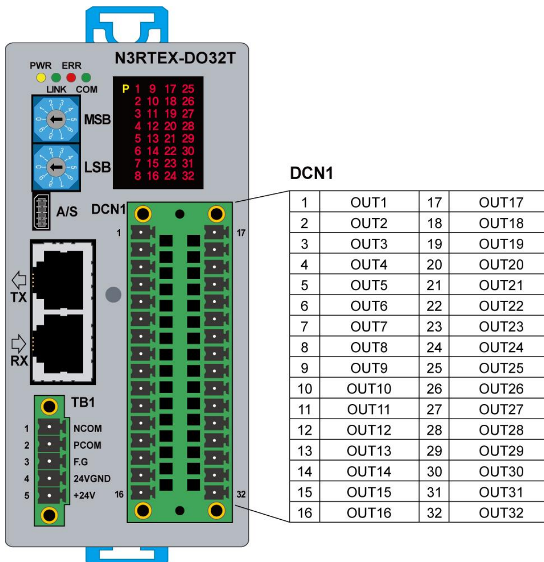
그림 21. N3RTEX-DO32T 모듈 DCN1 커넥터 핀 배열
