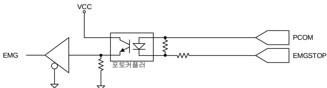
그림 72. N3RTEX-PM2Q/PM4Q 모듈의 비상정지 회로 구성도
