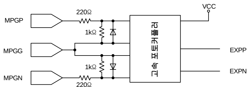
그림 70. N3RTEX-PM2Q/PM4Q 모듈의 MPG 입력 회로 구성도
