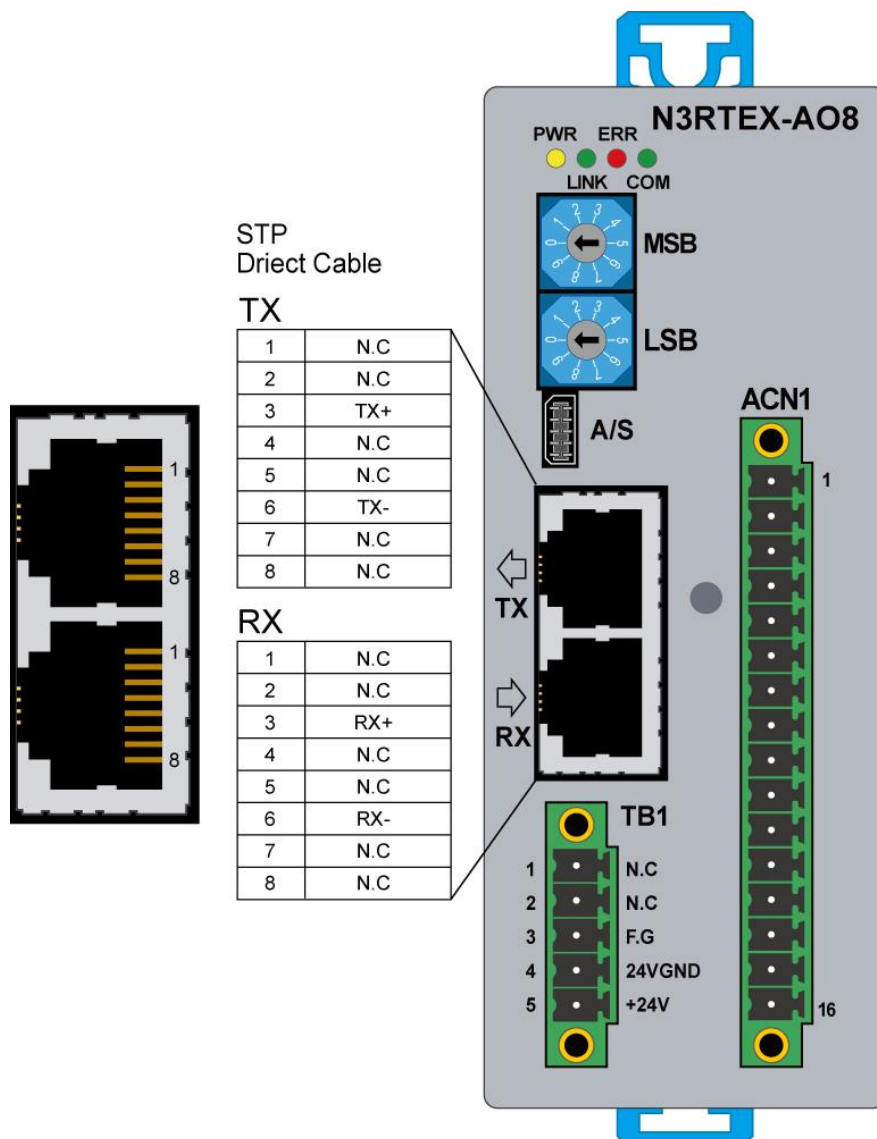
그림 40. N3RTEX-AO8 모듈 RTEX 통신 커넥터 핀 배열 (RX, TX)
