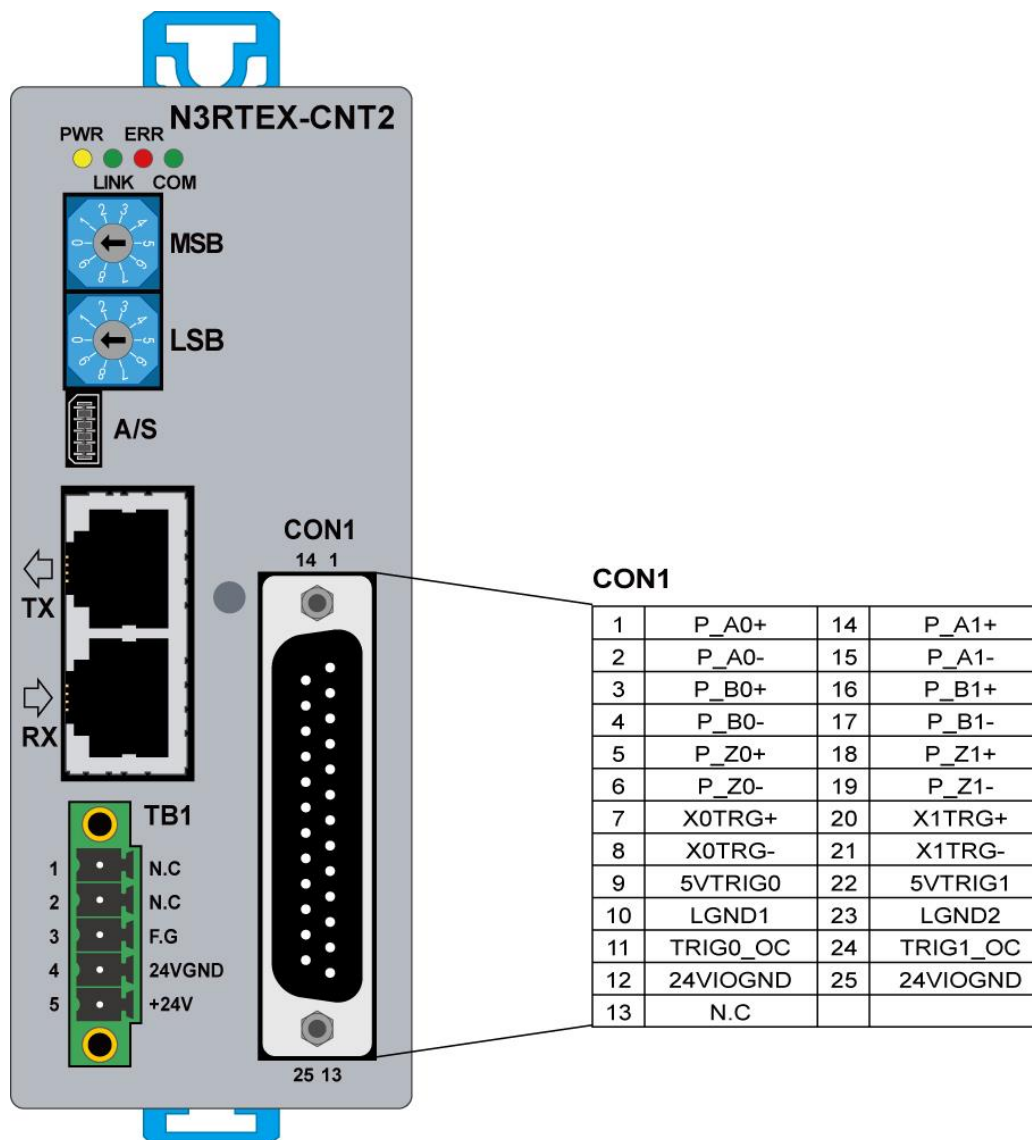
그림 52. N3RTEX-CNT2 커넥터 핀 배열
