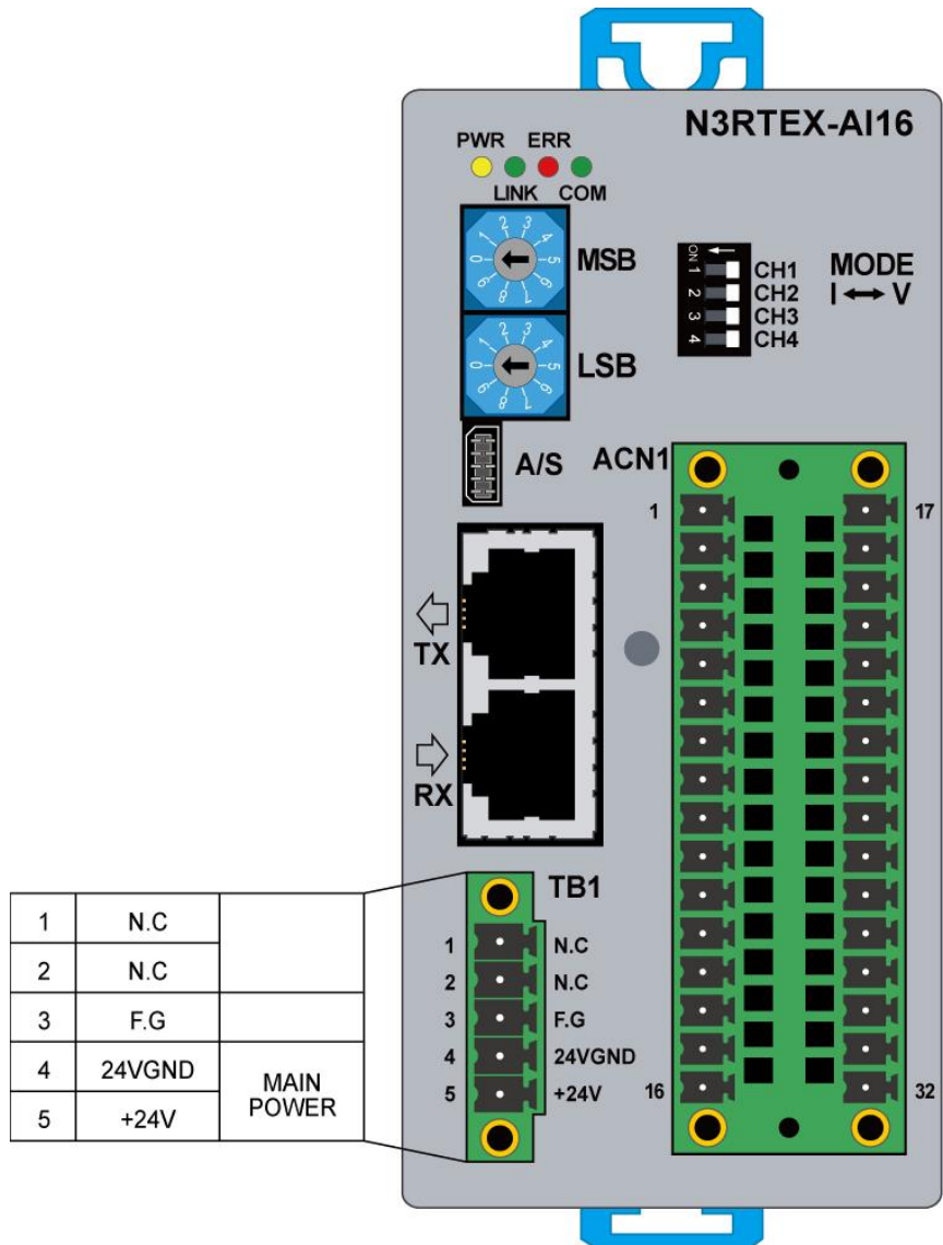
그림 36. N3RTEX-AI16 모듈 TB1 커넥터 핀 배열
