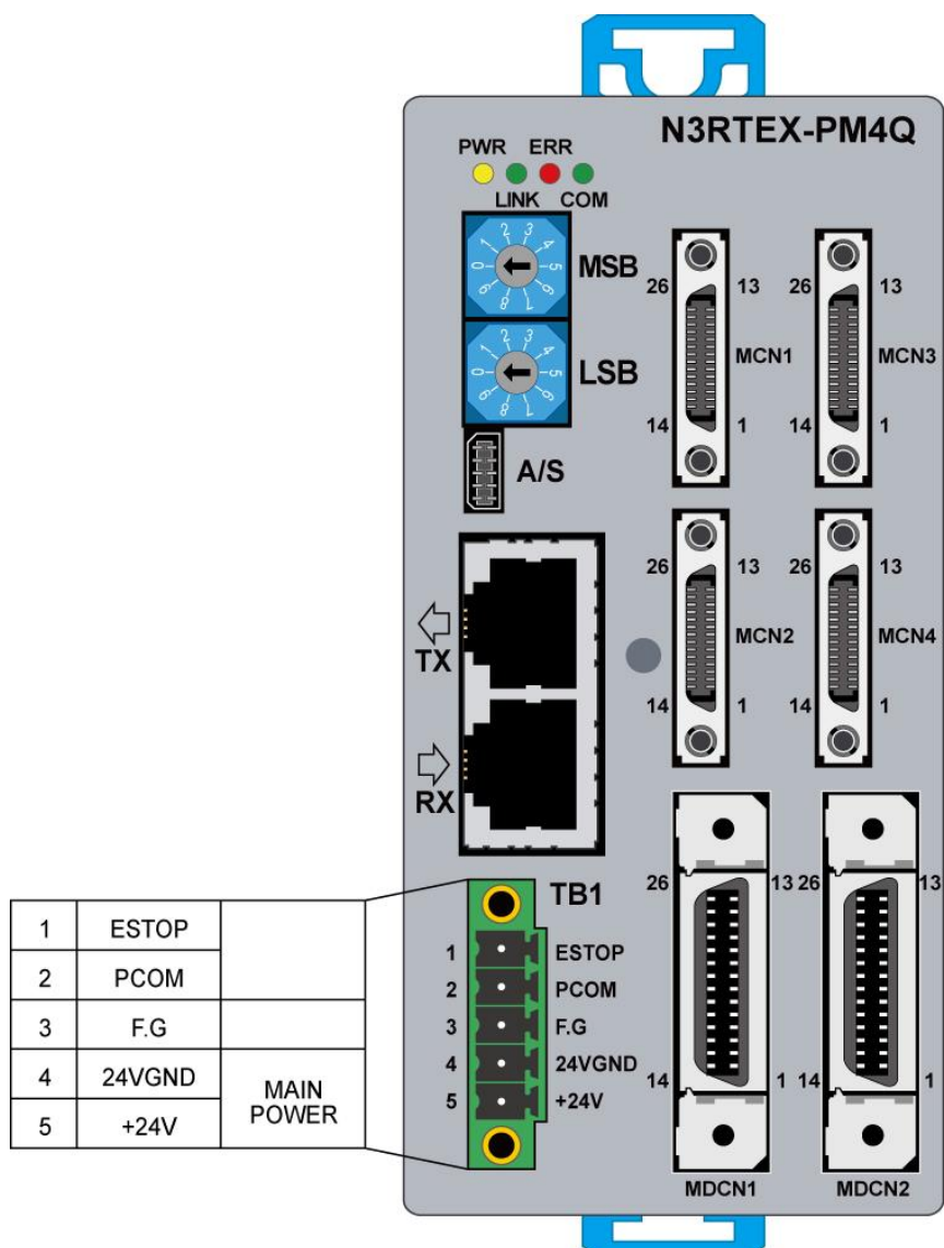
그림 51. N3RTEX-PM4Q 모듈 TB1 커넥터 핀 배열
