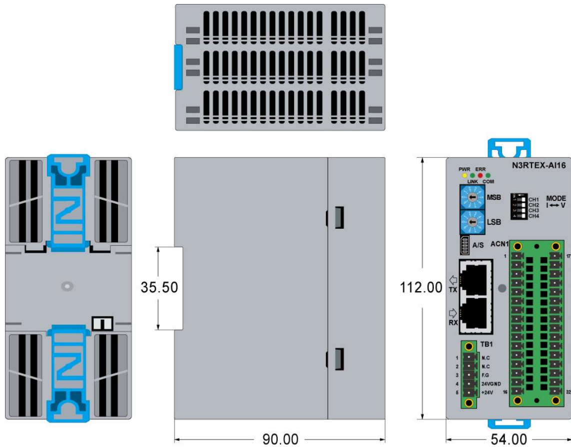
그림 8. N3RTEX-AI16 모듈의 사이즈 및 형상
