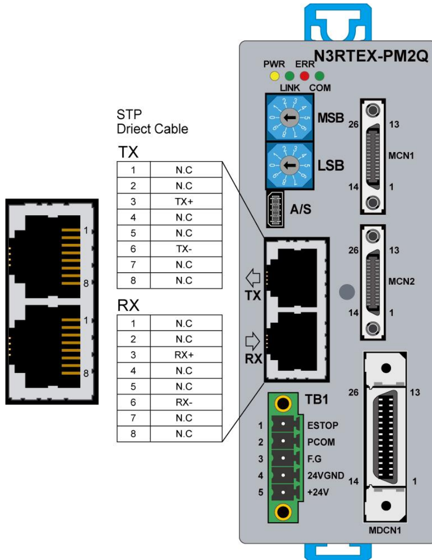
그림 45. N3RTEX-PM2Q 모듈 RTEX 통신 커넥터 핀 배열 (RX, TX)
