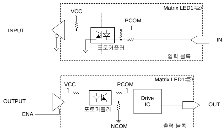
그림 61. N3RTEX-DB32T 모듈 내부의 디지털 입력/출력 회로 구성도
