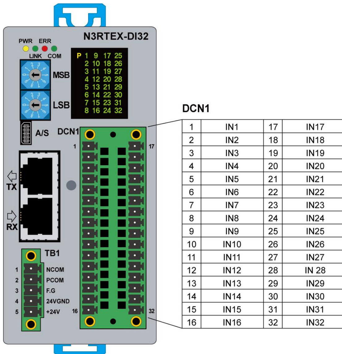
그림 16. N3RTEX-DI32 모듈 DCN1 커넥터 핀 배열
