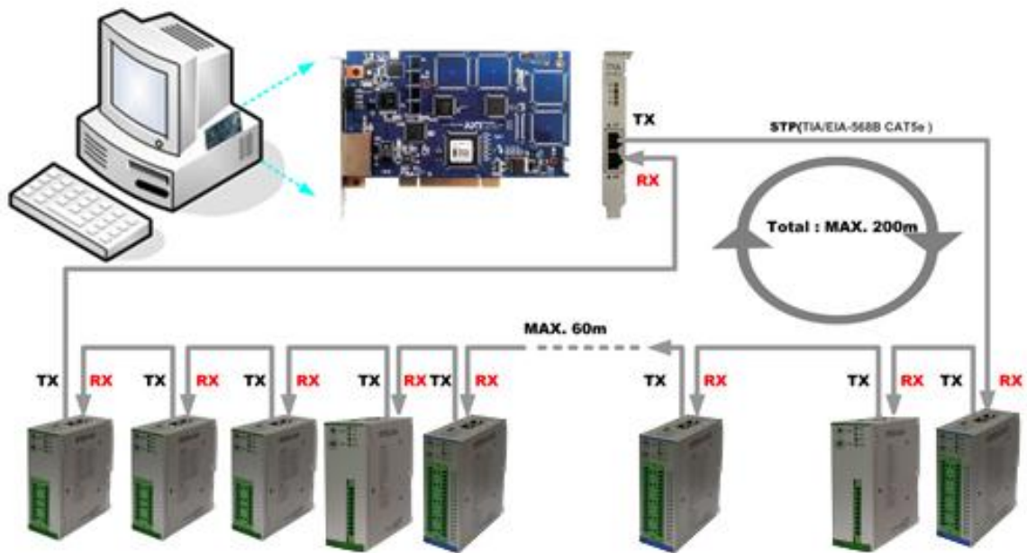
그림 4. RTEX 네트워크 연결도
