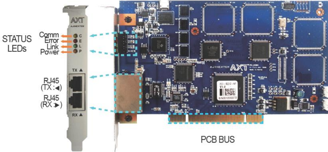
그림 3. PCI-R1604 RTEX master 보드와 커넥터
