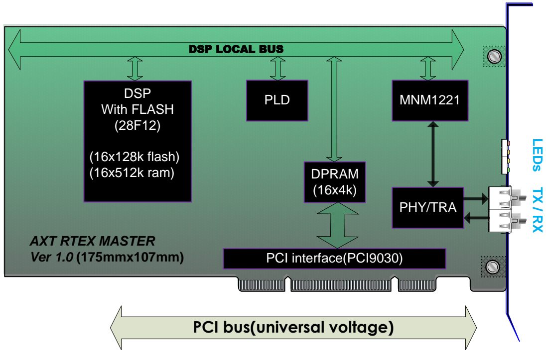
그림 2. PCI-R1604 블록도
