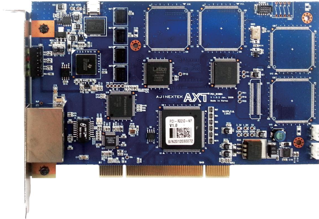
그림 1. PCI-R1604 실물 사진
