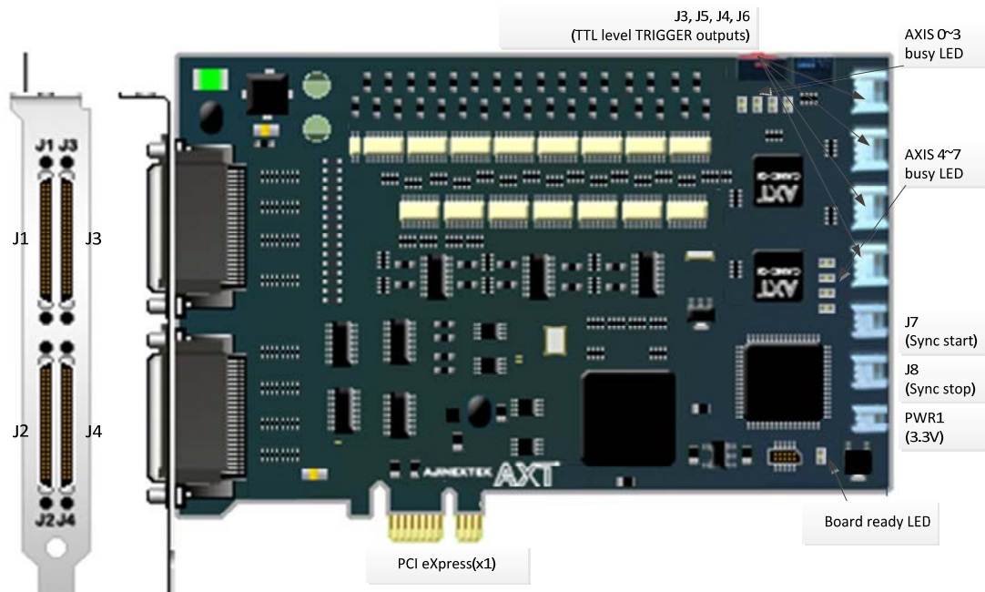
그림 3. PCIe-N804보드와 커넥터
