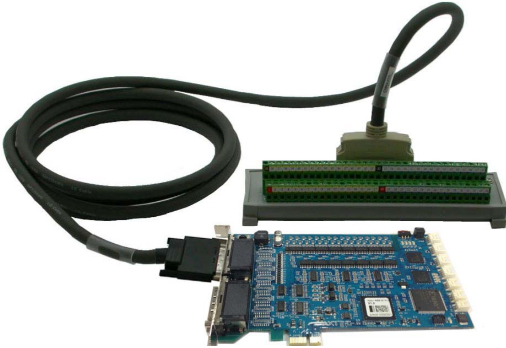
그림 13. PCIe-N804 보드와 단자대간의 결선 그림
