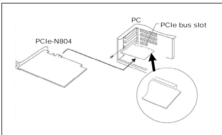
그림 1. PCI express 슬롯 장착 및 확인
