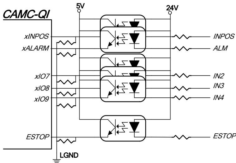
그림 9. INPOS, ALM, IN2, IN3, EMGN, SSTOP 인터페이스(X 축)
