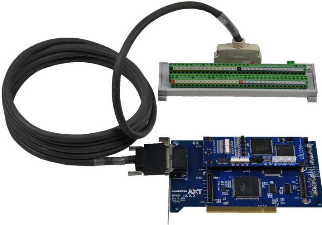
그림 12. SMC-2V04를 장착한 캐리어 보드와 단자대간의 결선 그림 (BPHR의 경우)
