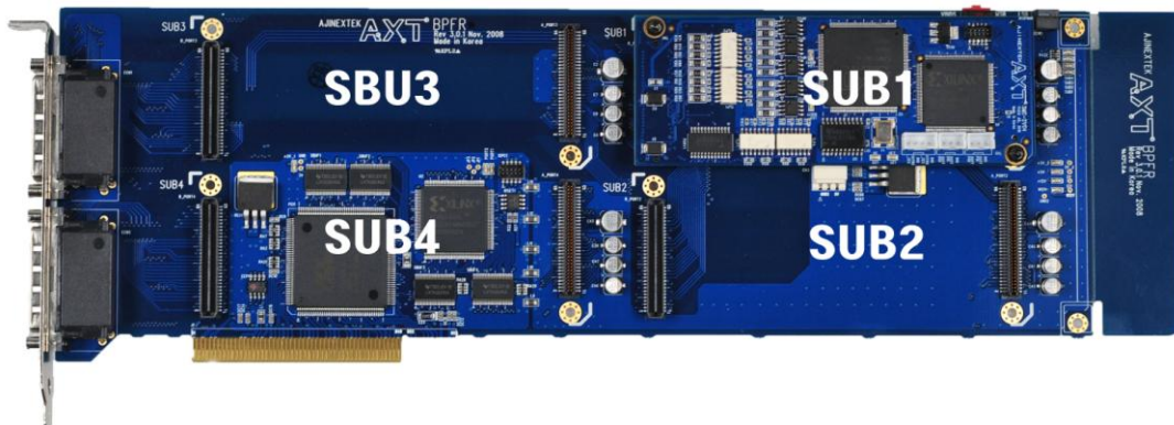
그림 18. BPFR에 장착된 SMC-2V04
