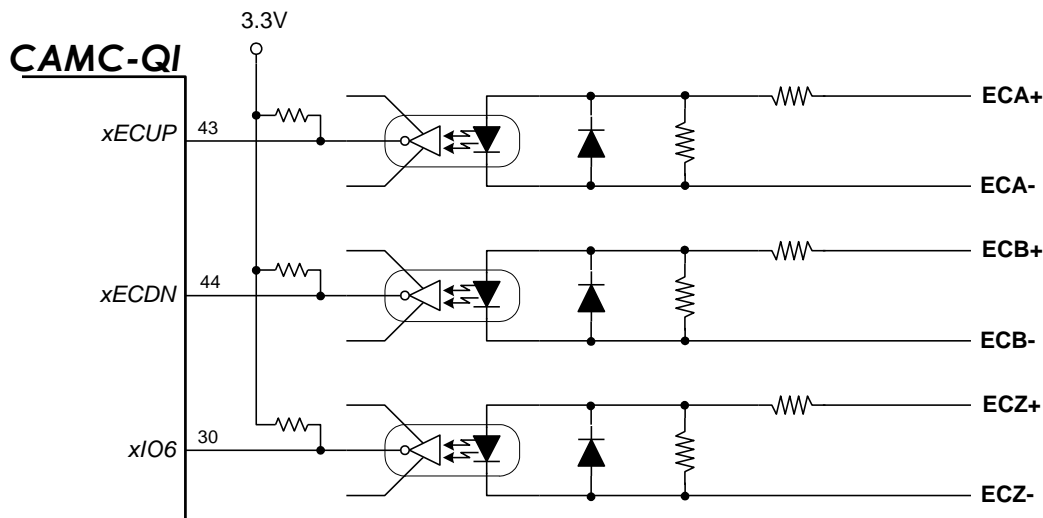
그림 9. 엔코더 A, B, Z상 신호의 인터페이스
