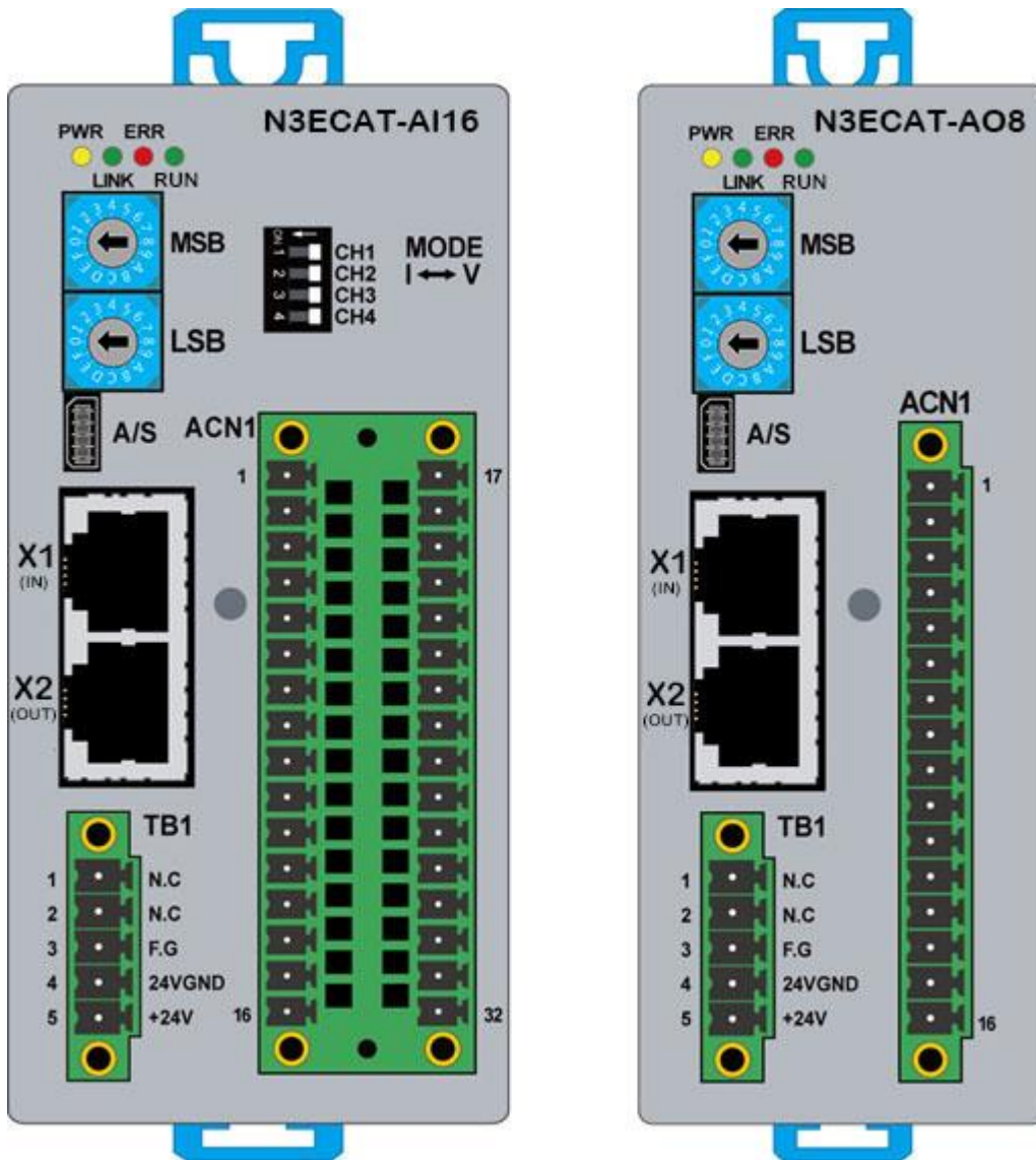
그림 1. N3 ECAT AIO SLAVE 모듈
