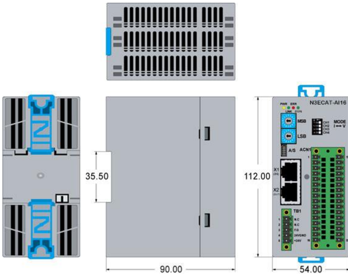
그림 2. N3ECAT-AI16 모듈의 사이즈 및 형상
