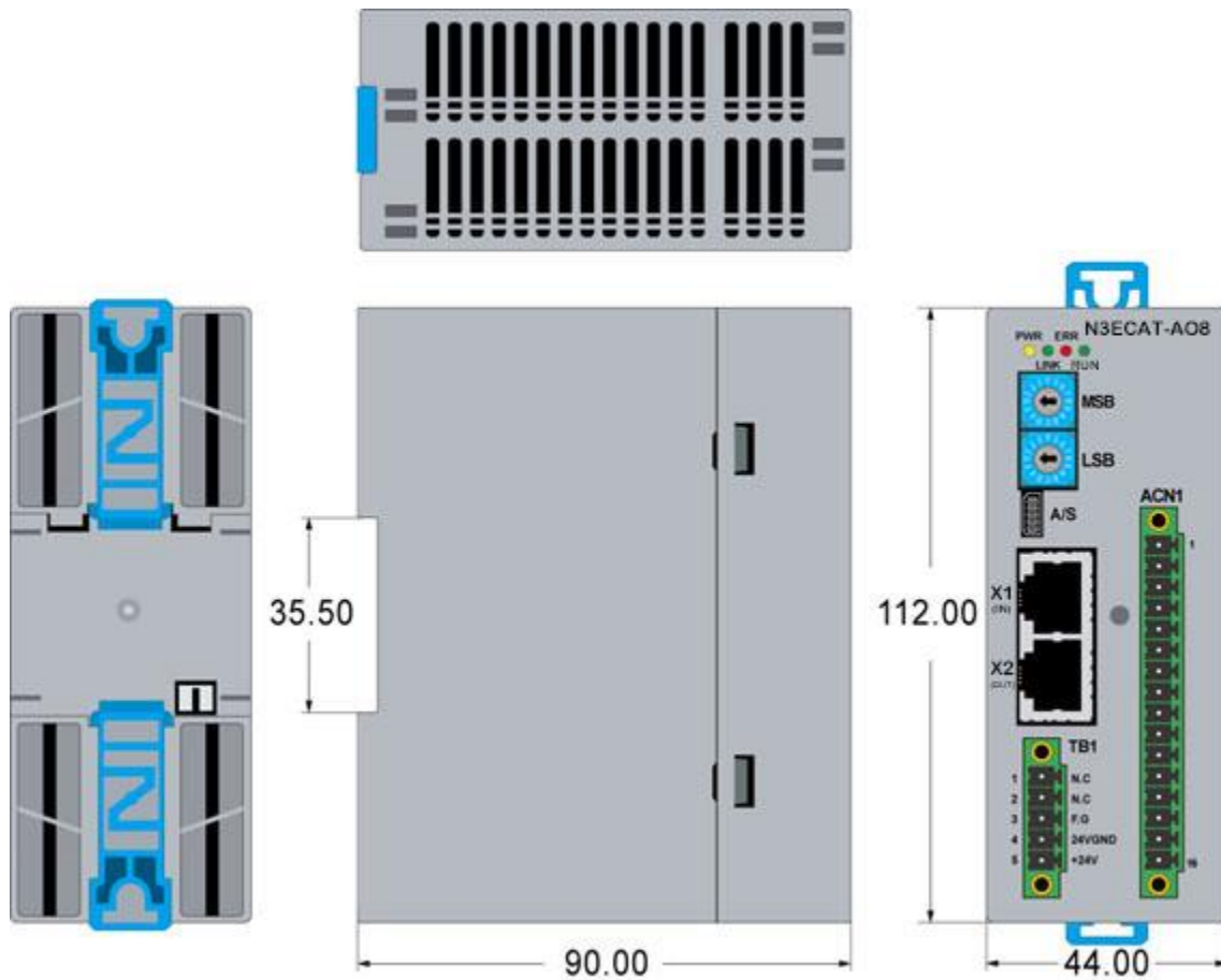
그림 3. N3RTEX-AO8 모듈의 사이즈 및 형상
