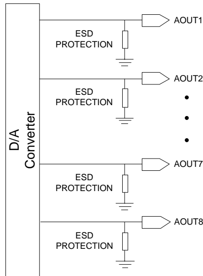
그림 20. N3ECAT-AO8 모듈 내부의 아날로그 출력 회로 구성도
