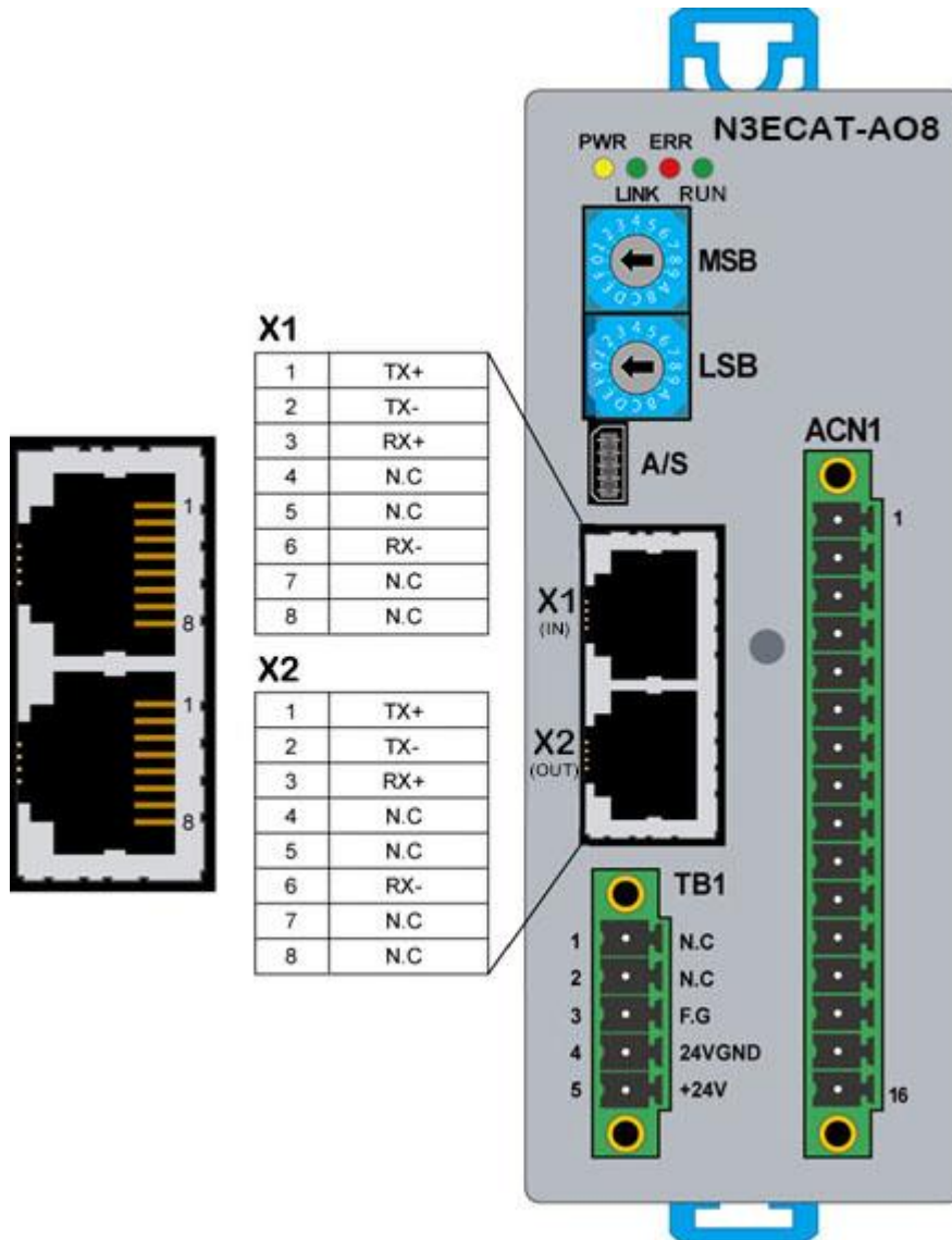
그림 16. N3ECAT-AO8 모듈 EtherCAT 통신 커넥터 핀 배열 (X1, X2)
