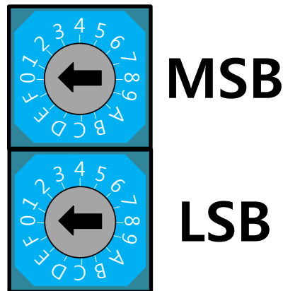
그림 10. N3ECAT-AI16 모듈 NODE ID 스위치
