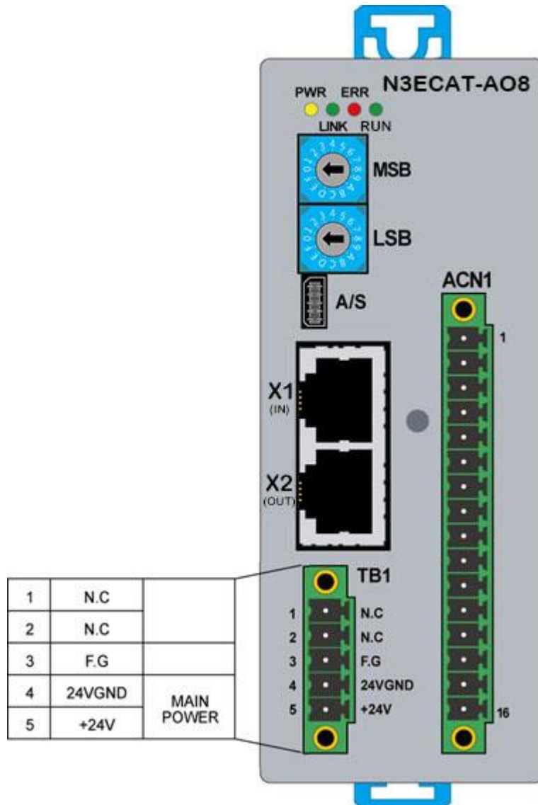
그림 17. N3ECAT-AO8 모듈 TB1 커넥터 핀 배열
