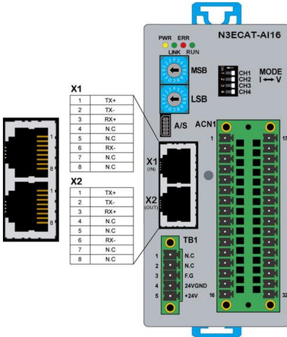
그림 11. N3ECAT-AI16 모듈 EtherCAT 통신 커넥터 핀 배열 (X1, X2)
