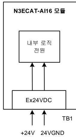
그림 19. N3ECAT-AI16 모듈 전원 회로 구성도
