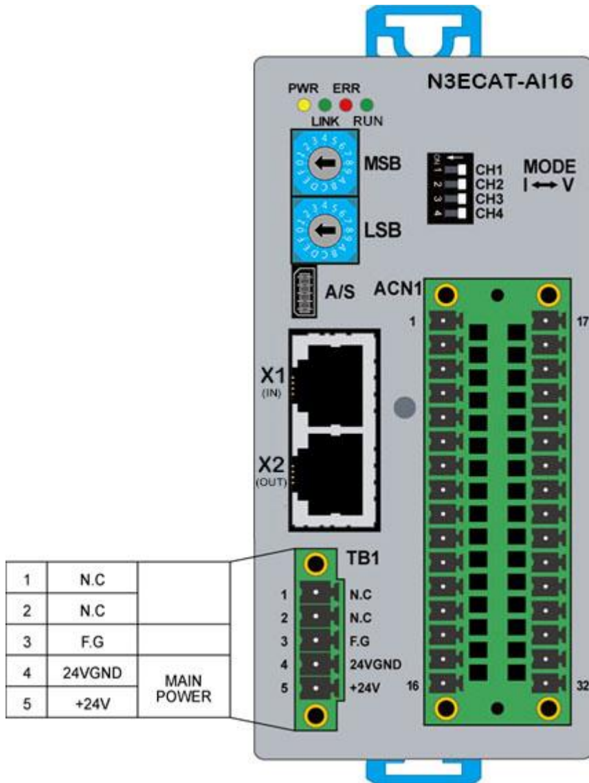
그림 12. N3ECAT-AI16 모듈 TB1 커넥터 핀 배열
