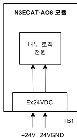
그림 21. N3ECAT-AO8 모듈 전원 회로 구성도
