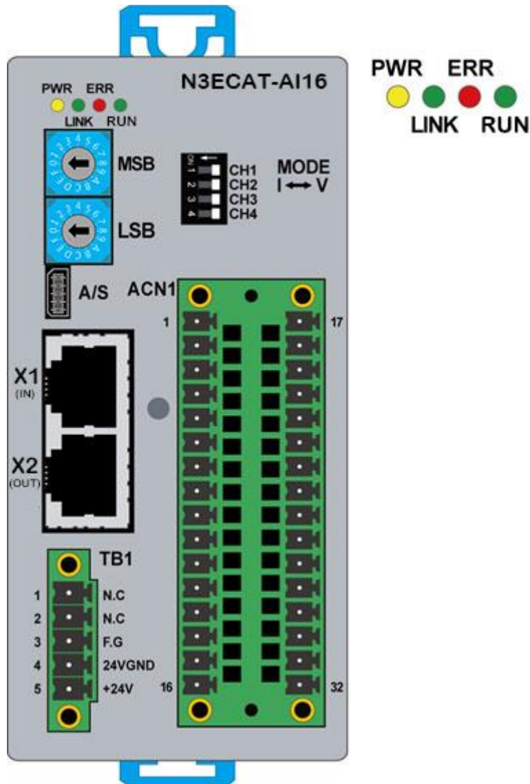
그림 8. N3ECAT-AI16 모듈 LED 표시부
