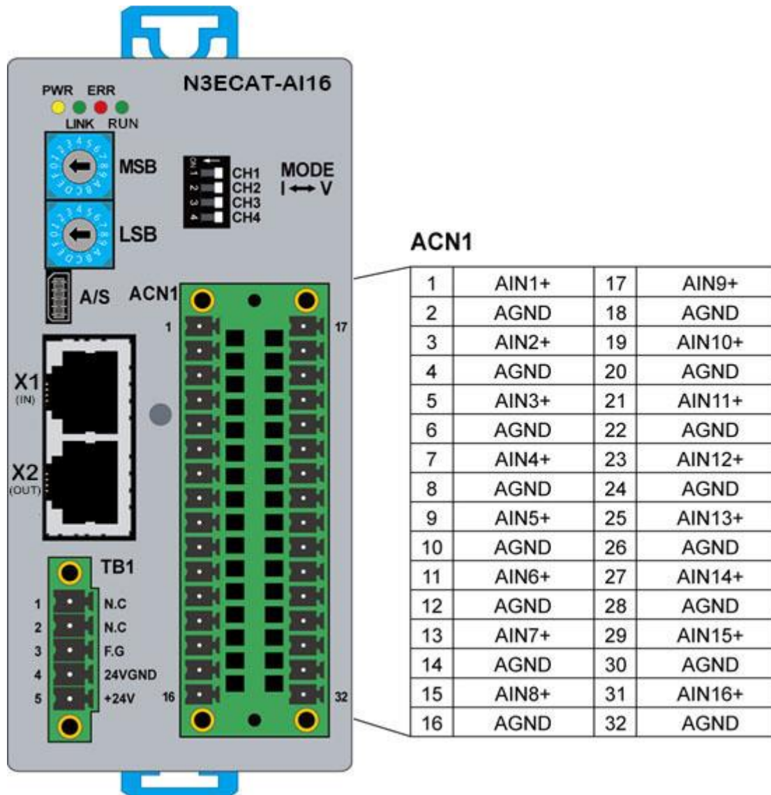
그림 7. N3ECAT-AI16 모듈 ACN1 커넥터 핀 배열
