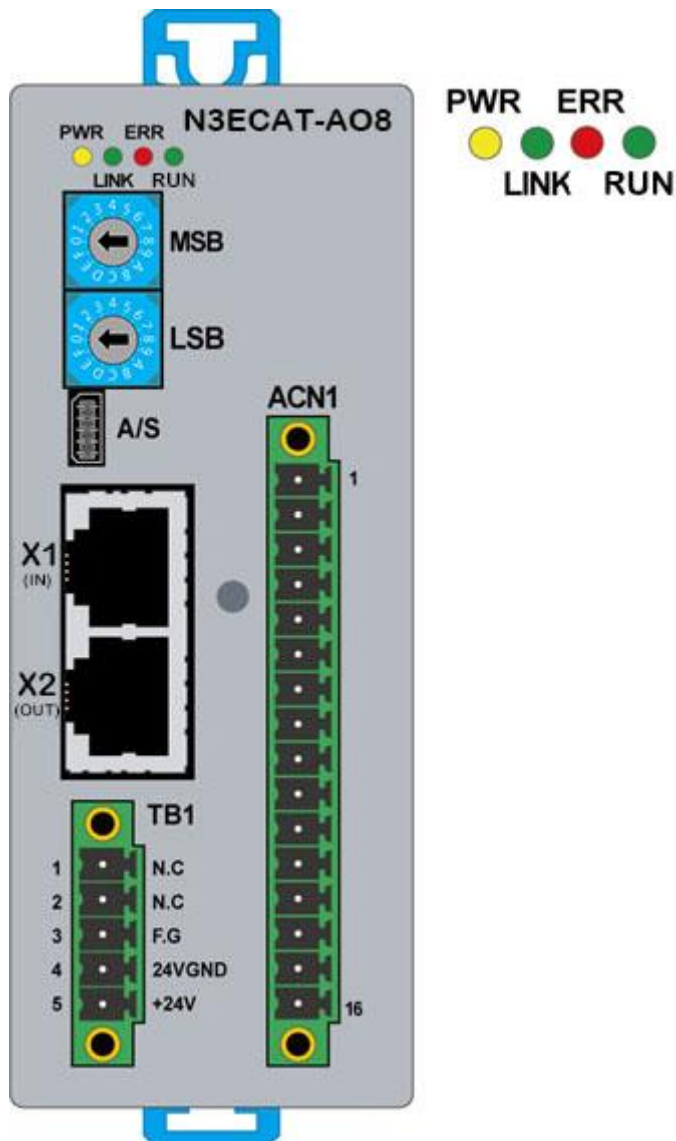
그림 14. N3ECAT-AO8 모듈 LED 표시부
