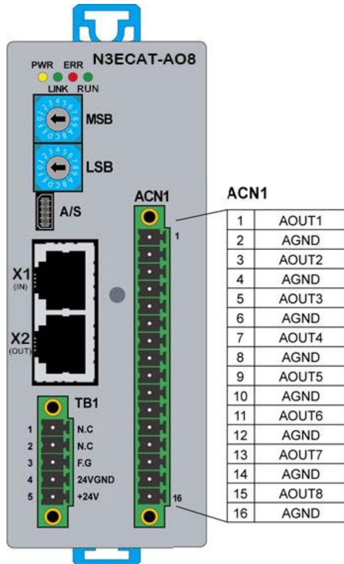
그림 13. N3ECAT-AO8 모듈 ACN1 커넥터 핀 배열
