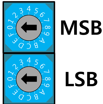
그림 15. N3ECAT-AO8 모듈 NODE ID 스위치
